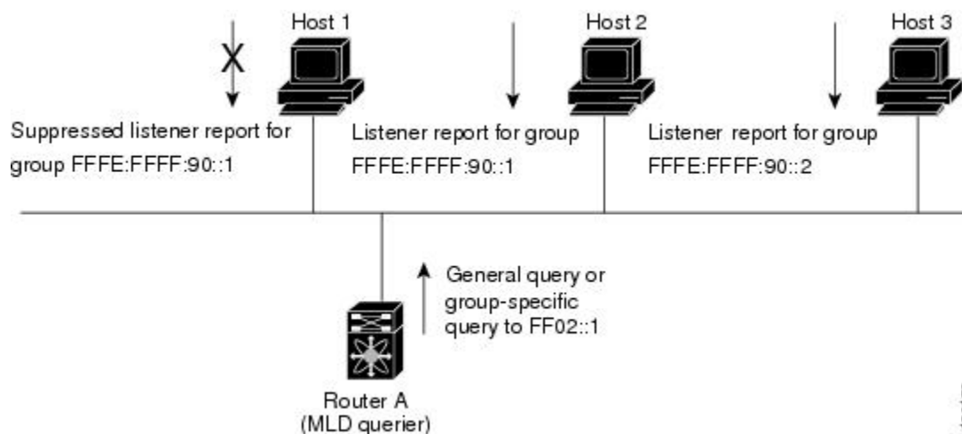
図 1: MLD クエリー応答プロセス
