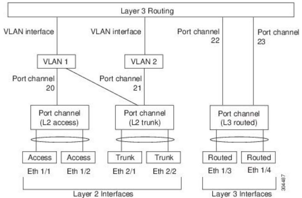
図 9: ポートチャネルインターフェイス
