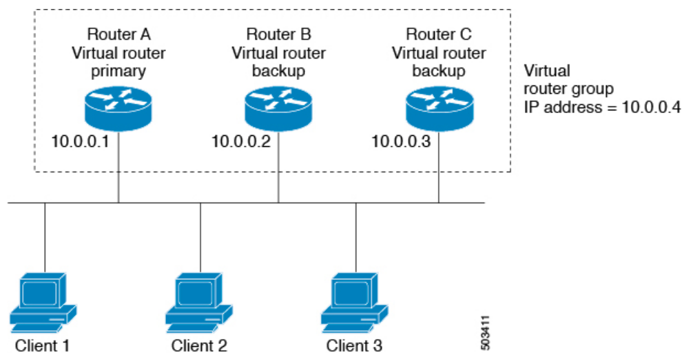
図 1: 基本的な VRRP トポロジ
