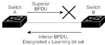
Figure 7: 単方向リンク障害の検出
