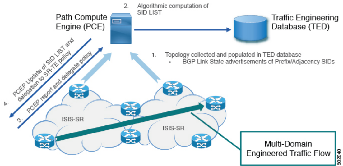
図 8: ODN 操作
