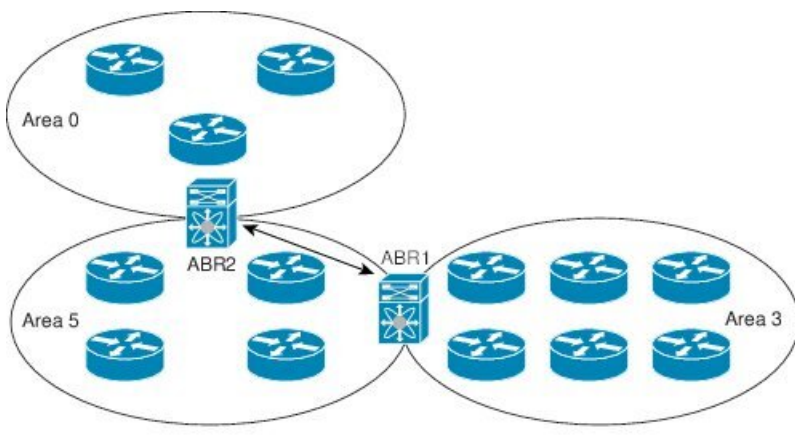
図 4: 仮想リンク
