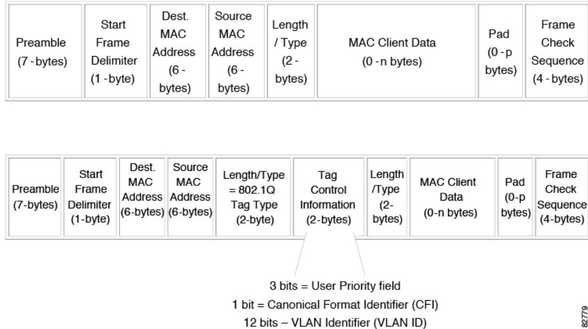
Figure 2: 802.1Q タグが含まれているヘッダーと含まれていないヘッダー
