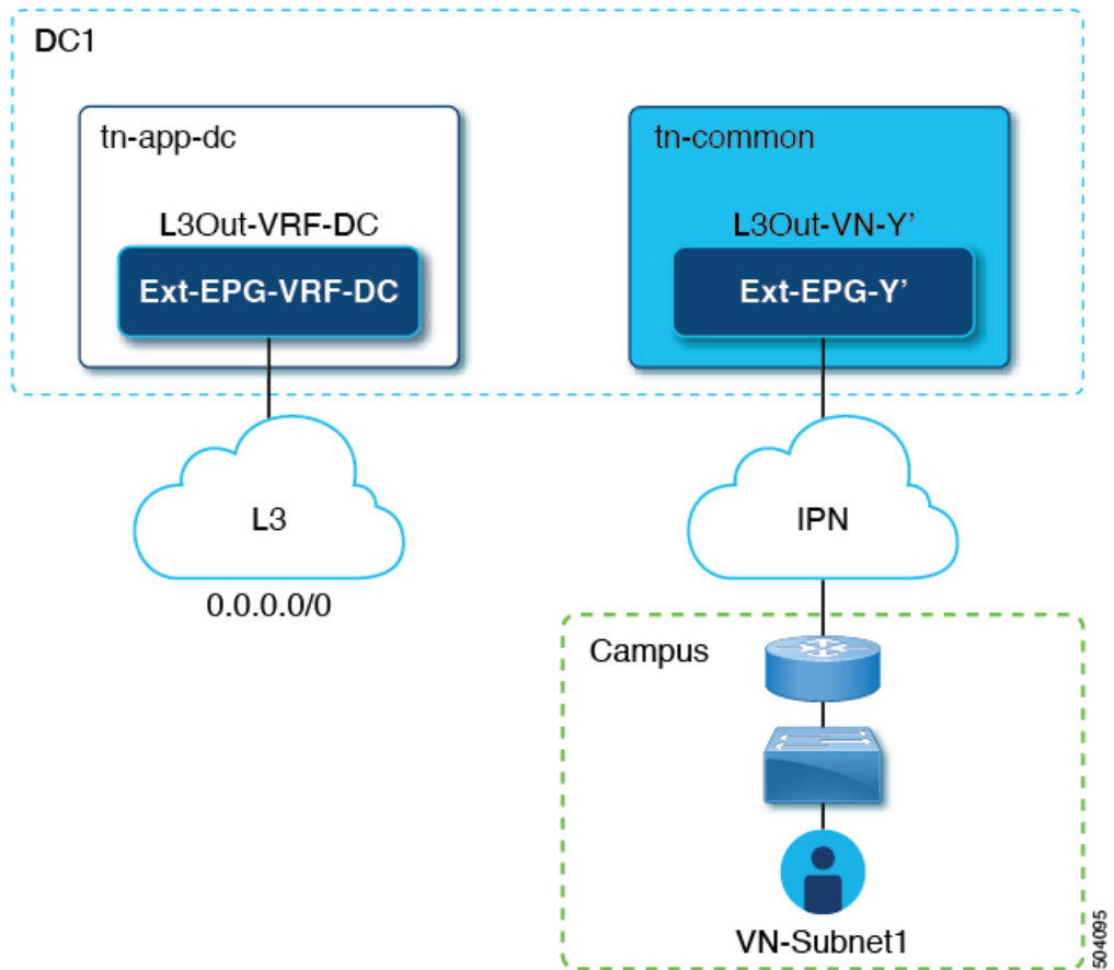
図 5: L3Out 接続
