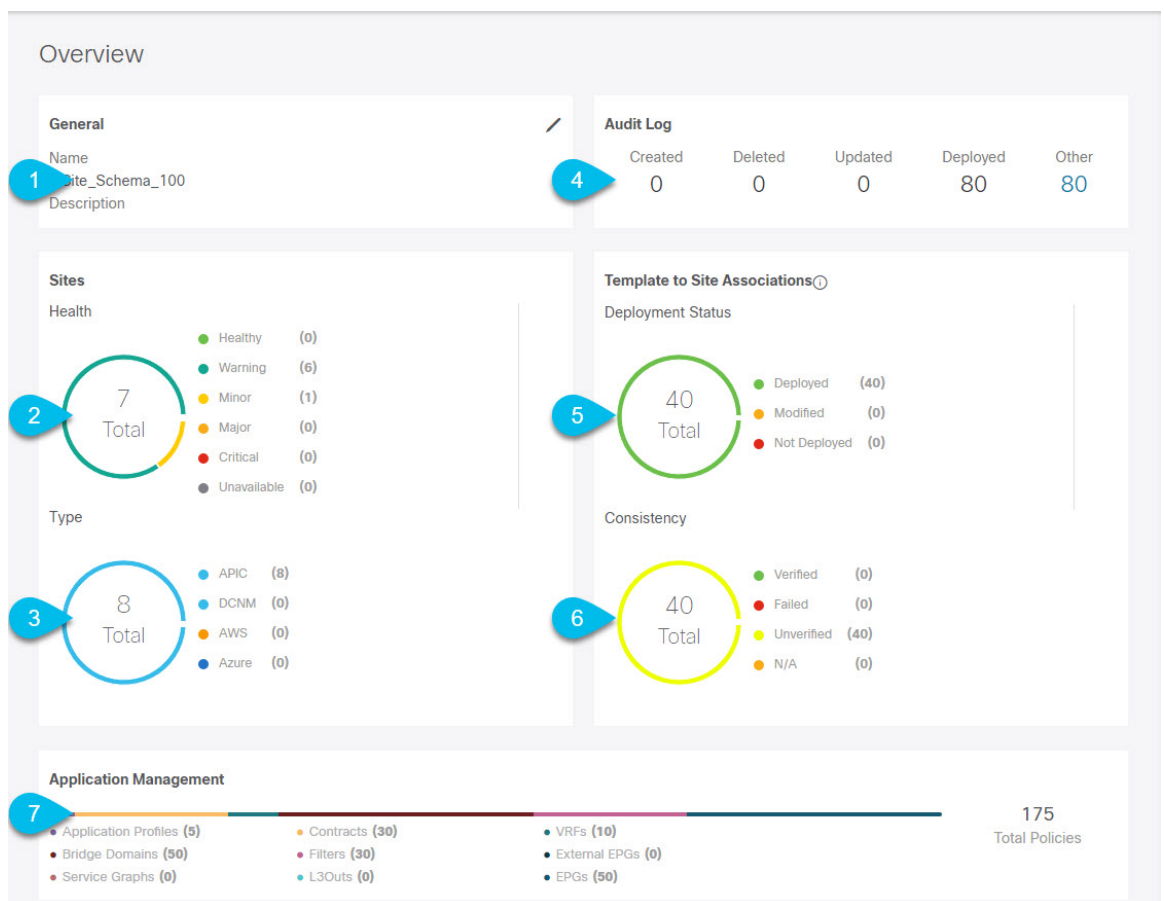
図 6: スキーマの概要
