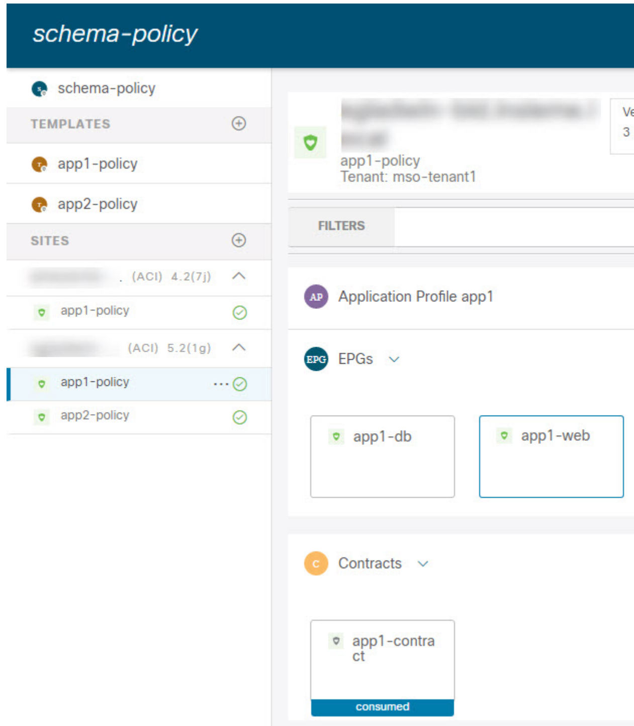
図 3: ポリシー スキーマ
