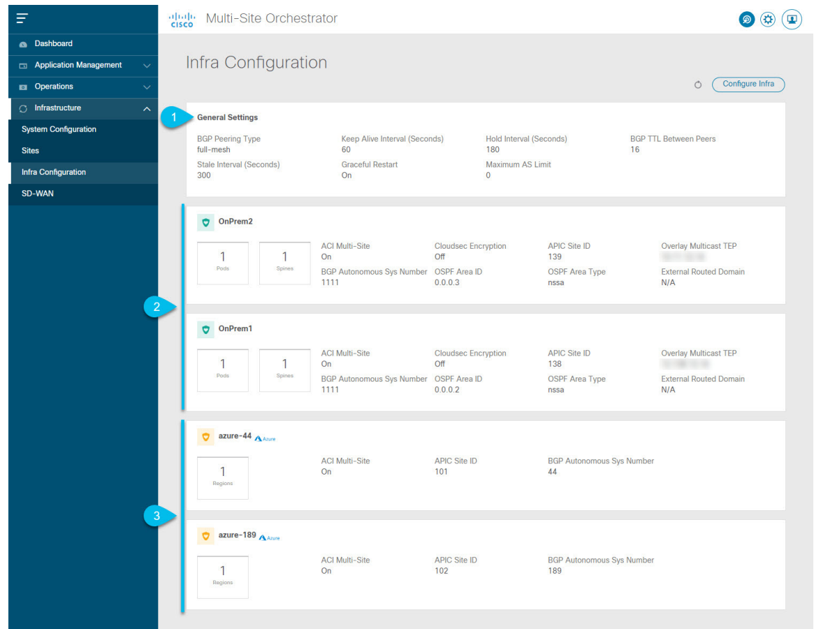
図 15: インフラ設定の概要
