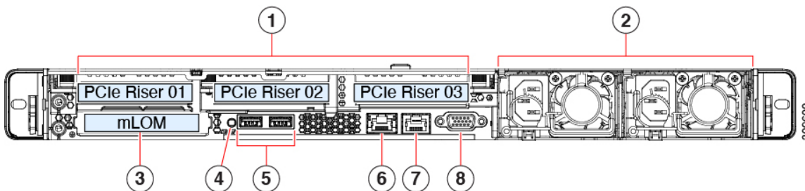
図 19 : Cisco ND-NODE-L4 背面パネルの 3 ライザーの構成
