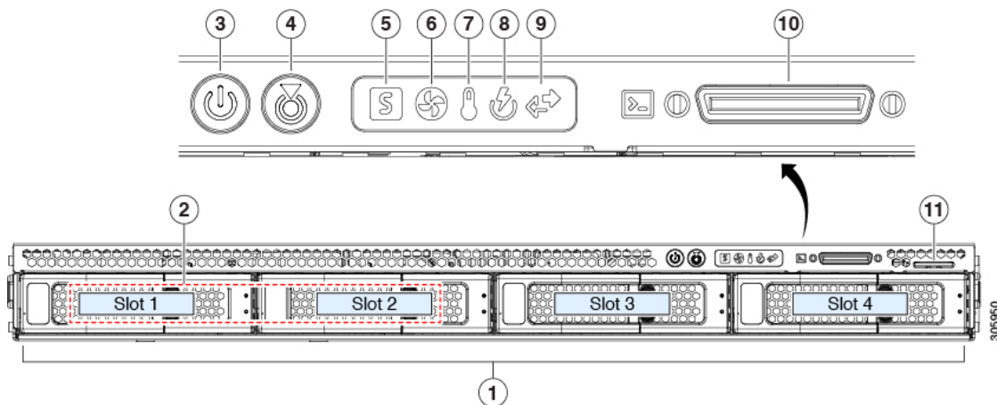
図 25: 31SE-CL-L3 (LFFドライブ) 前面パネルの機能
