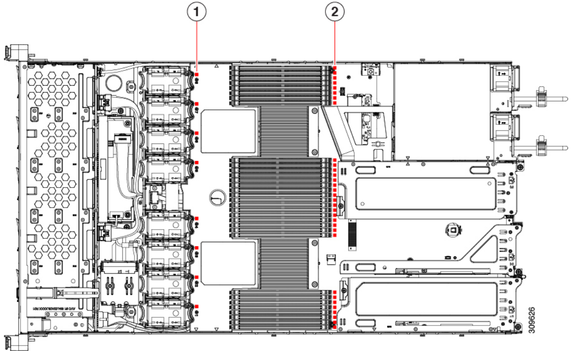
図 22: 内部診断 LED の位置
