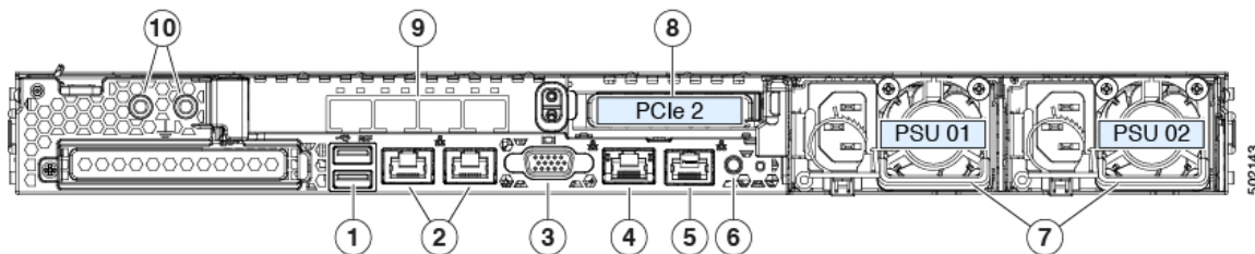
図 26: SE-CL-L3 背面パネル
