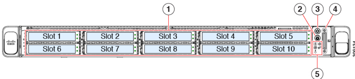
図 12: ND-NODE-G5S 前面パネル
