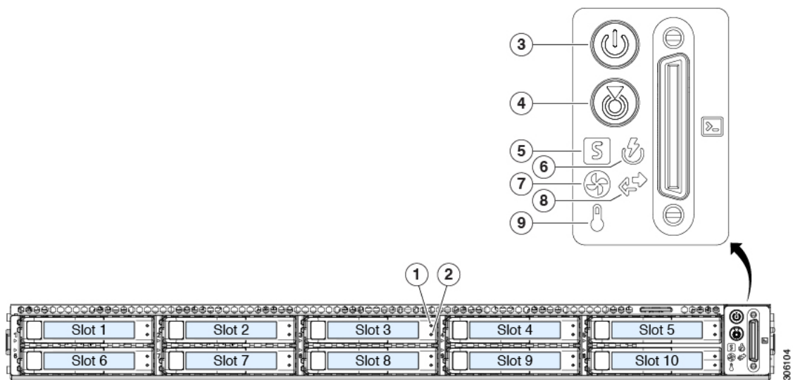
図 28: 前面パネルの LED
