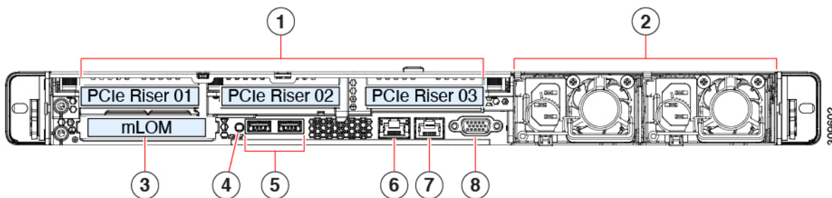
図 7: ND-NODE-G5L 背面パネルの 3 ライザーの構成
