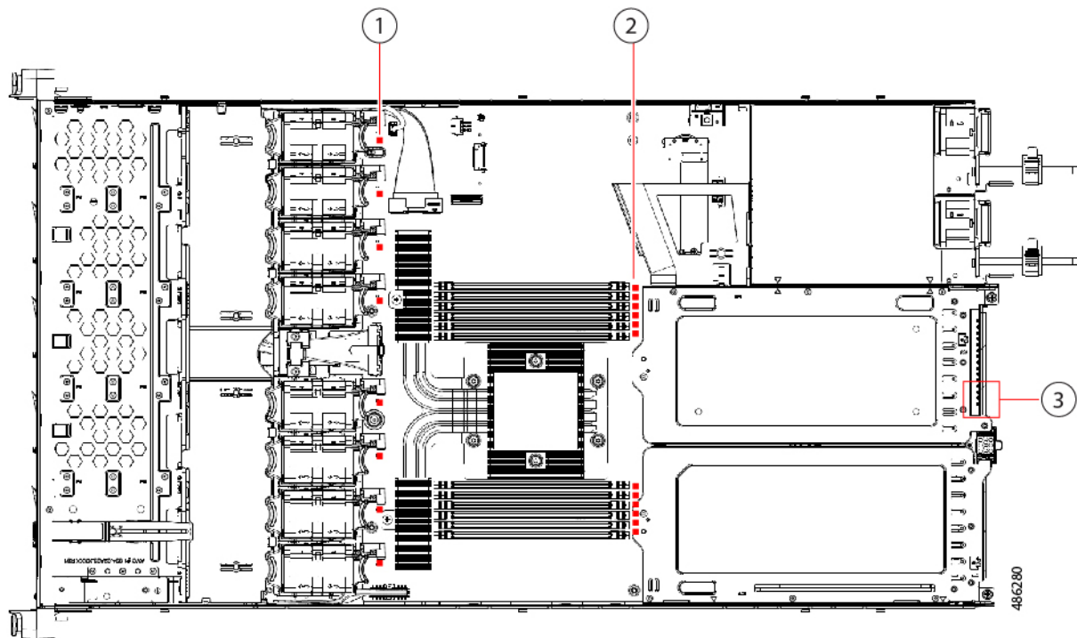
図 16: 内部診断 LED の位置
