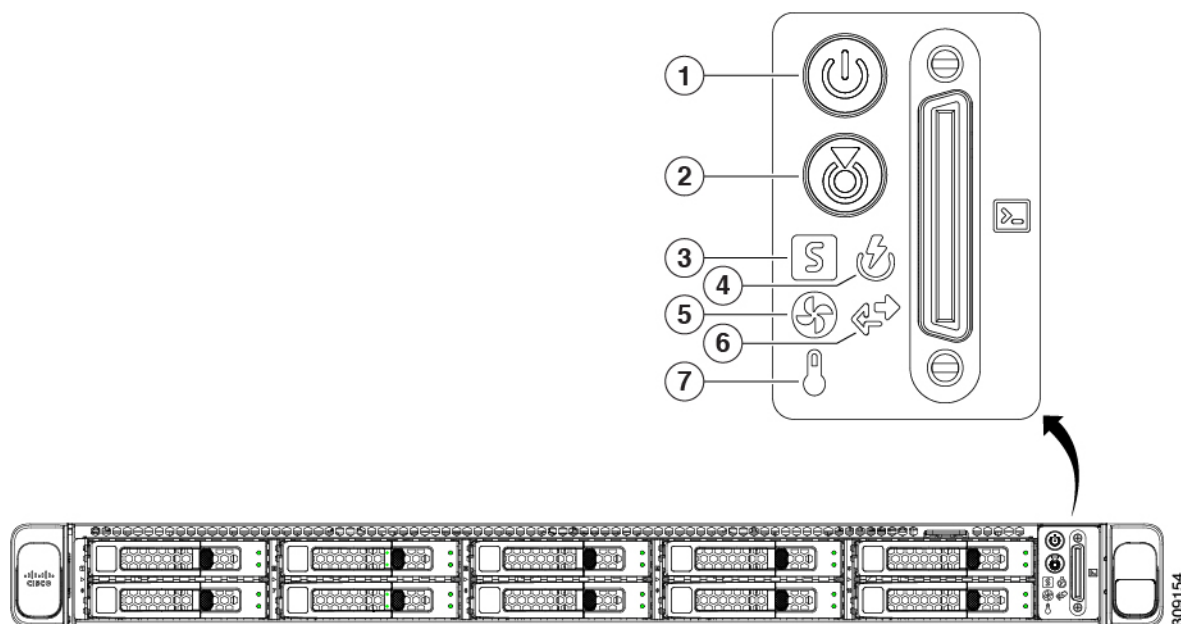
図 14: 前面パネルの LED
