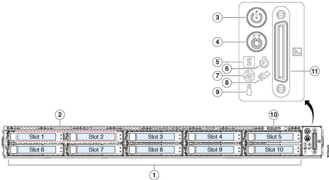
図 24: Cisco SE-CL-L3 (SFF ドライブ) 前面パネルの機能
