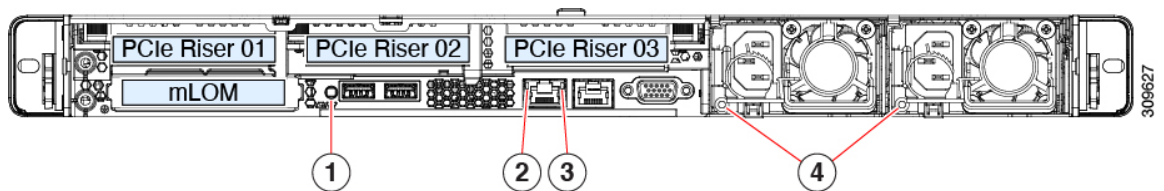
図 21: 背面パネル LED
