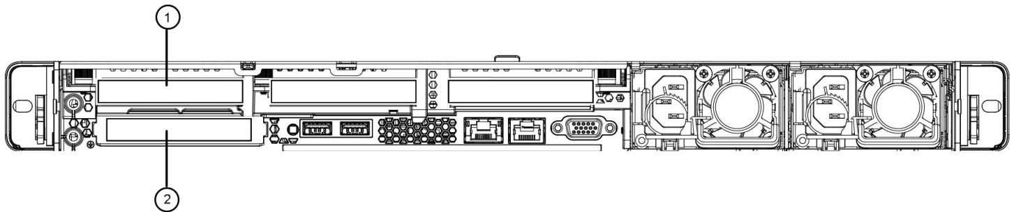
図 11: ノード接続に使用される mLOM および PCIe ライザー 01 カード : ND-NODE-G5L (UCS-C225-M8)
