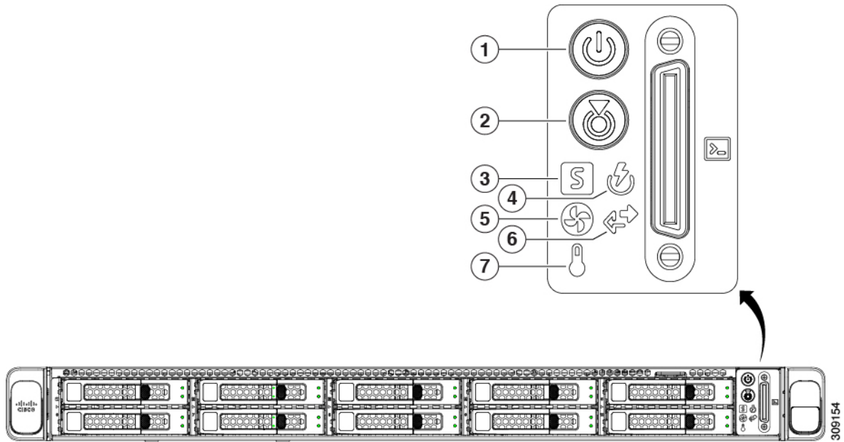
図 8: 前面パネルの LED
