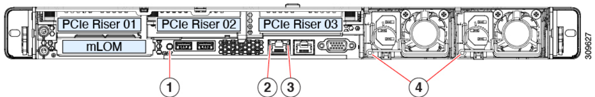
図 9: 背面パネル LED
