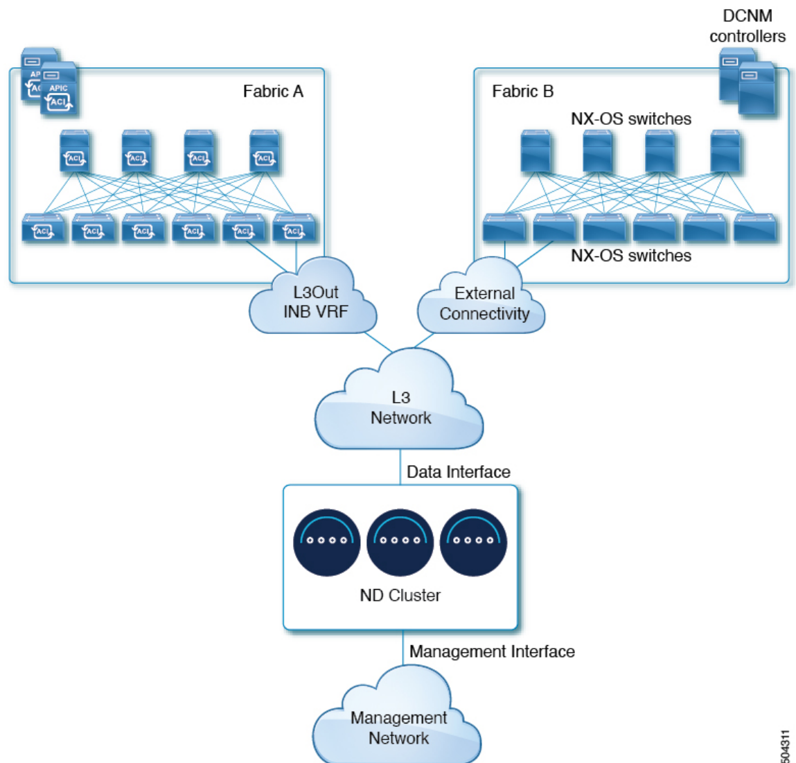
図 1: レイヤ 3 ネットワークを介した接続、2 日目の運用アプリケーション
