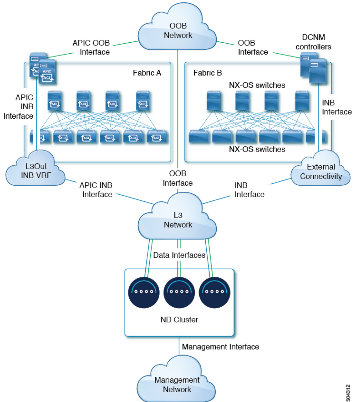
図 2: レイヤ3ネットワーク、 Nexus Dashboard Orchestrator を介した接続
