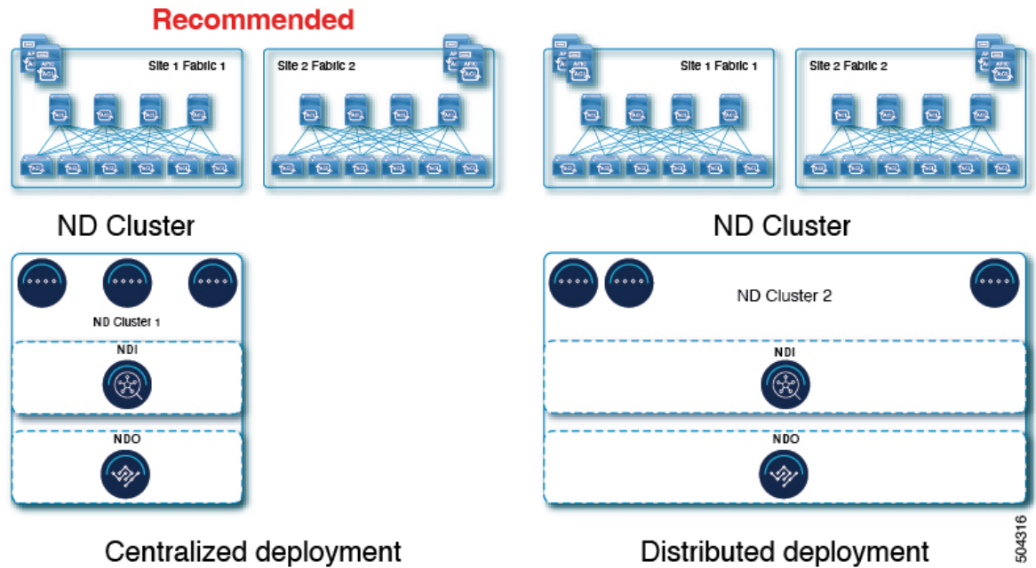
図 7: Nexus Dashboard Insights および Orchestrator の複数ファブリック、単一クラスタ
