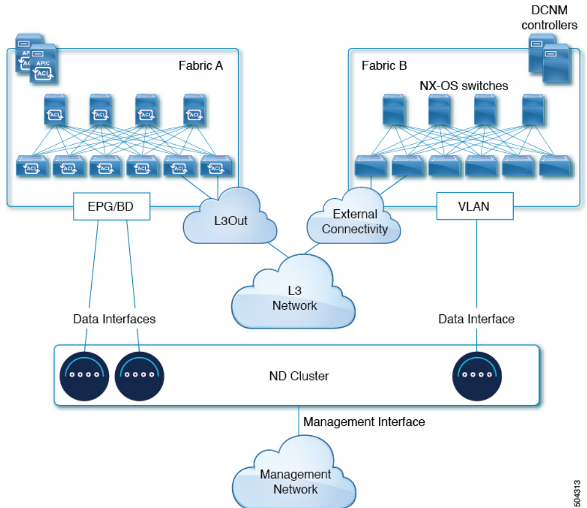
図 3: リーフスイッチへの直接接続、2日目の運用アプリケーション
