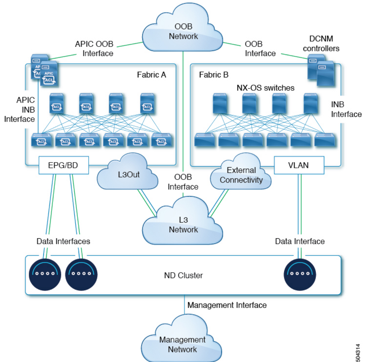
図 4: リーフスイッチ、Nexus ダッシュボードオーケストレータへの直接接続
