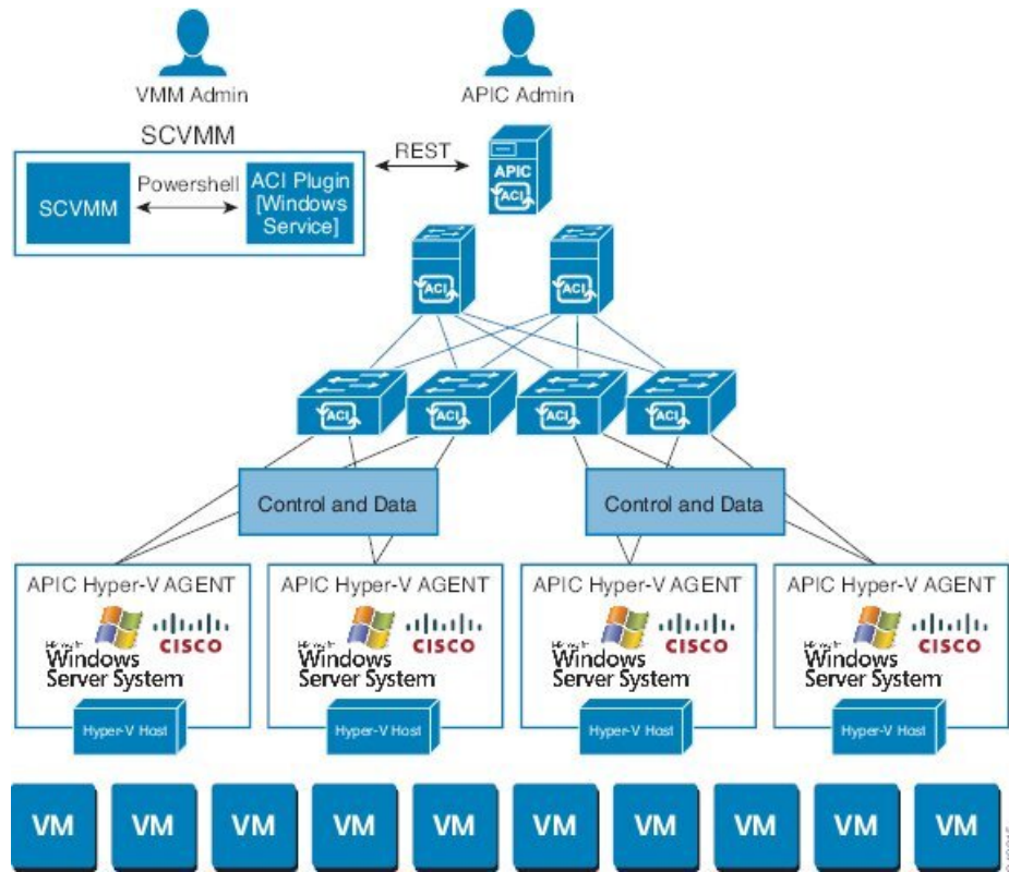
図 1: ACI ファブリックと SCVMM のトポロジ
