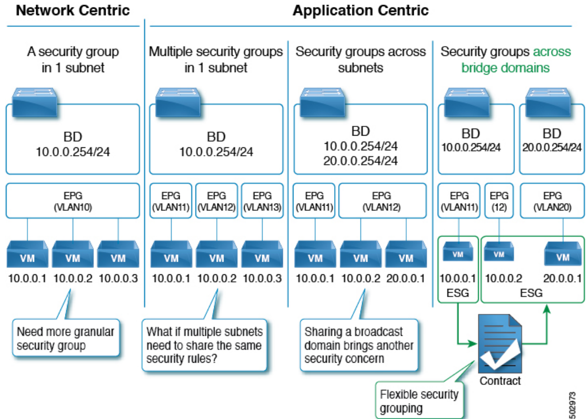
図 6: Cisco ACI では、複数のセグメンテーション オプションを提供します
