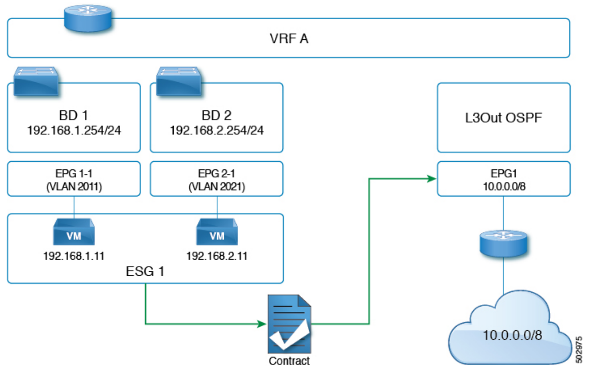
図 8: ESG から外部への接続は、L3 外部 EPG を使用して実装されます。
