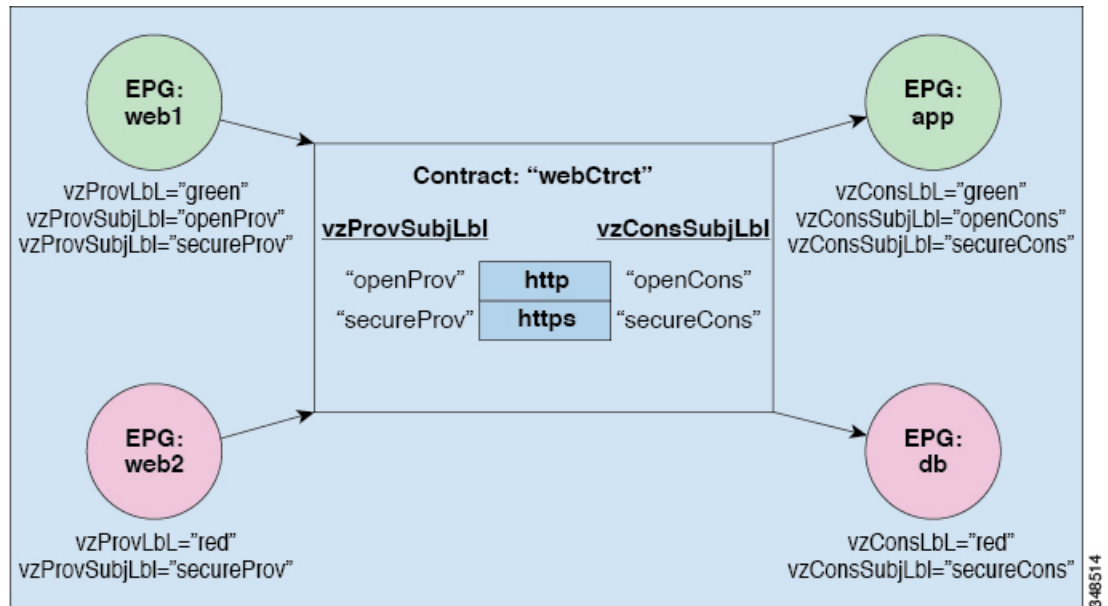
図 19: EPG/EPG 通信を決定するコントラクト
