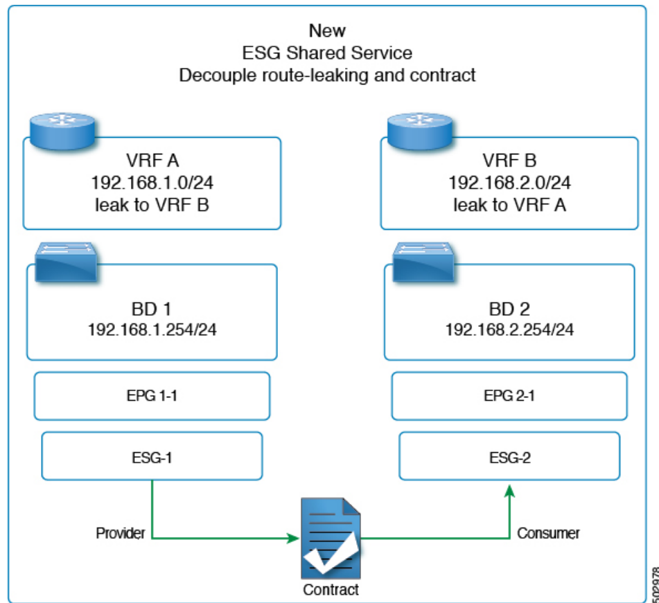
図 11: ESG によるルートリーク
