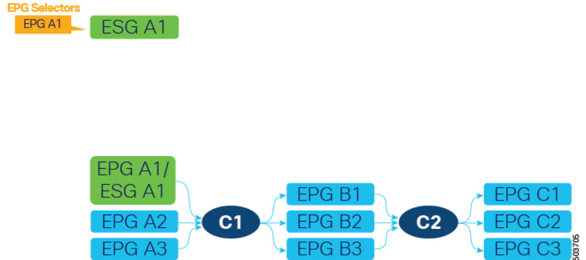
図 13: ESG を作成し、最初の EPG を移行します
