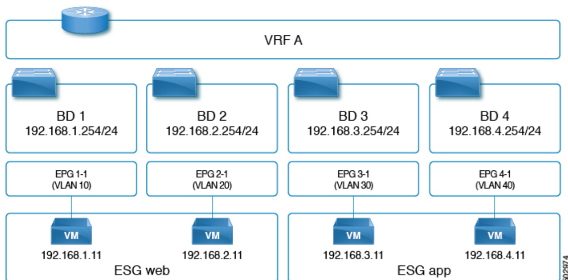
図 7: ESG を使用して、異なるサブネットのエンドポイントを集約できます
