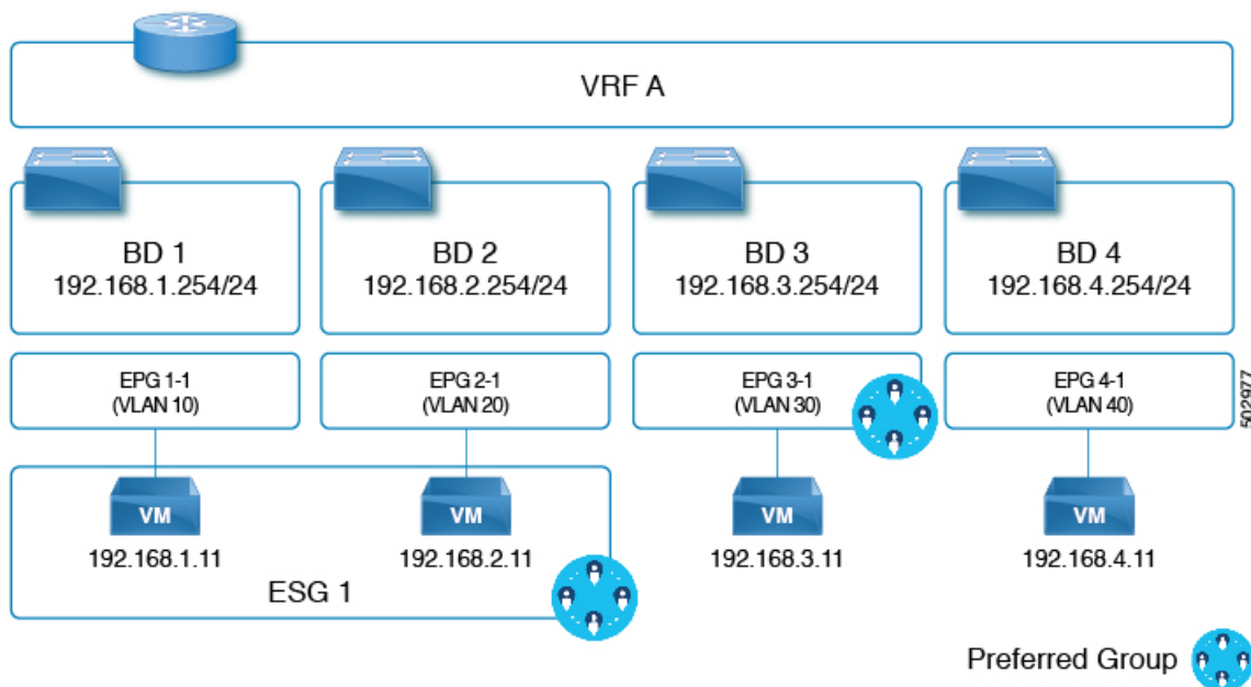
図 10: 同じ優先グループの ESG1 および EPG3-1 部分の例。
