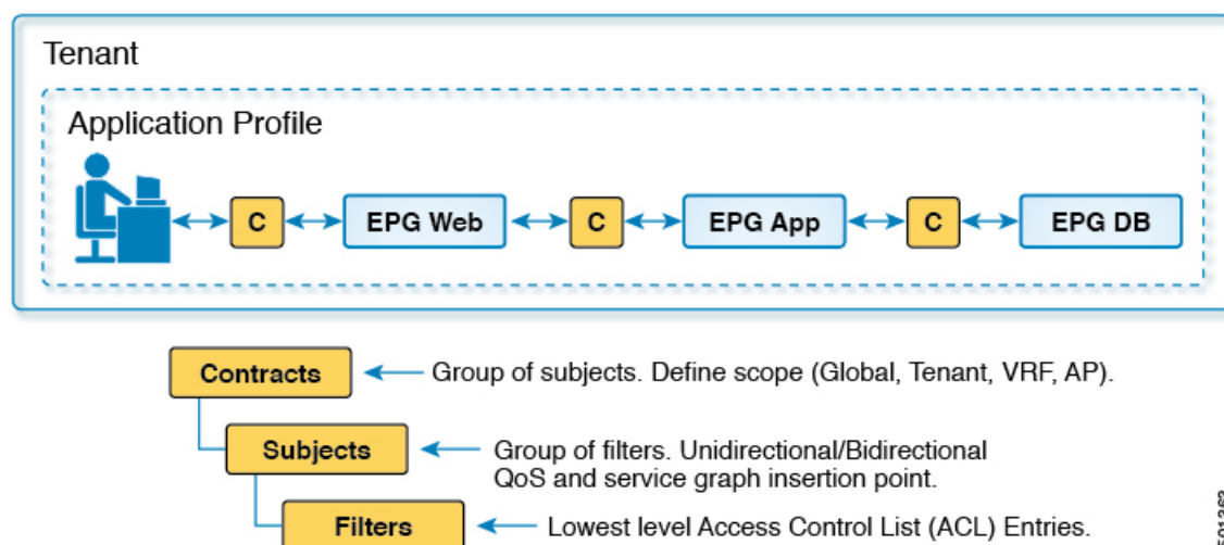
図 17: 契約のコンポーネント
