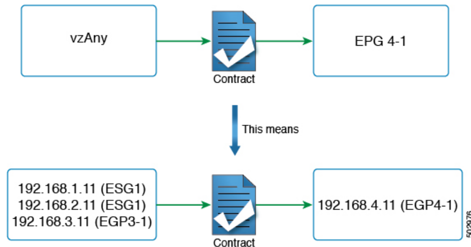
図 9: vzAny は、同じ VRF インスタンス内のすべての EPG と ESG を表す省略形です。
