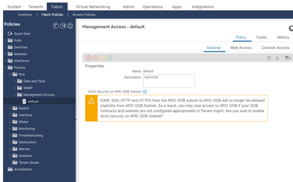
図 1: 厳密セキュリティ モードを有効にした後に表示される警告
