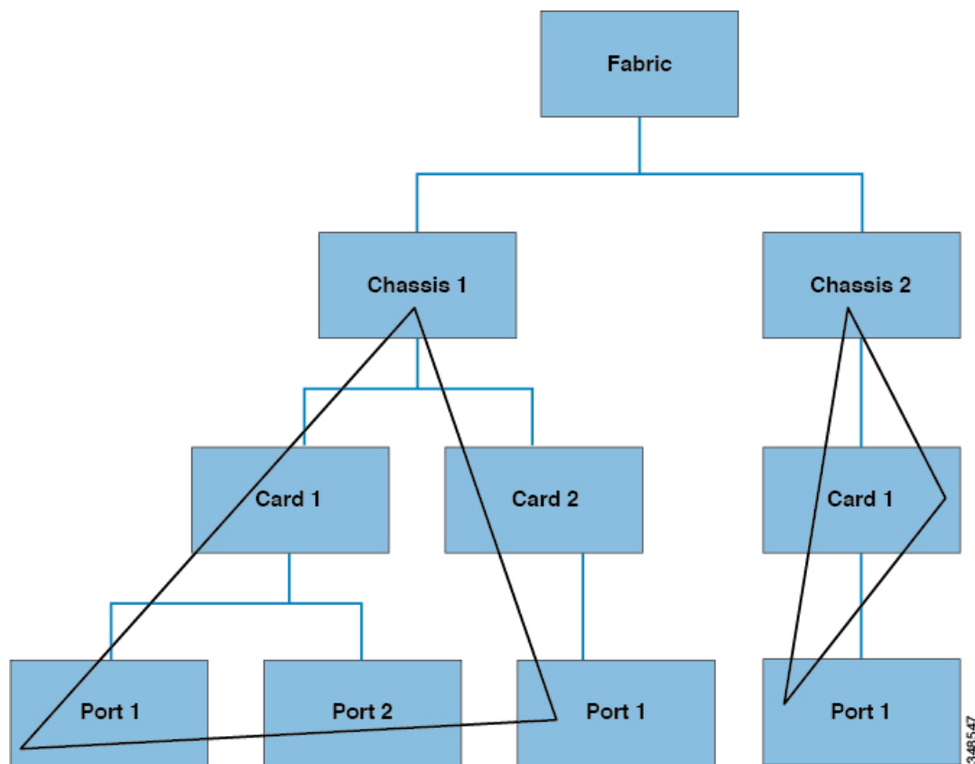
図 6: ツリーレベルのクエリ
