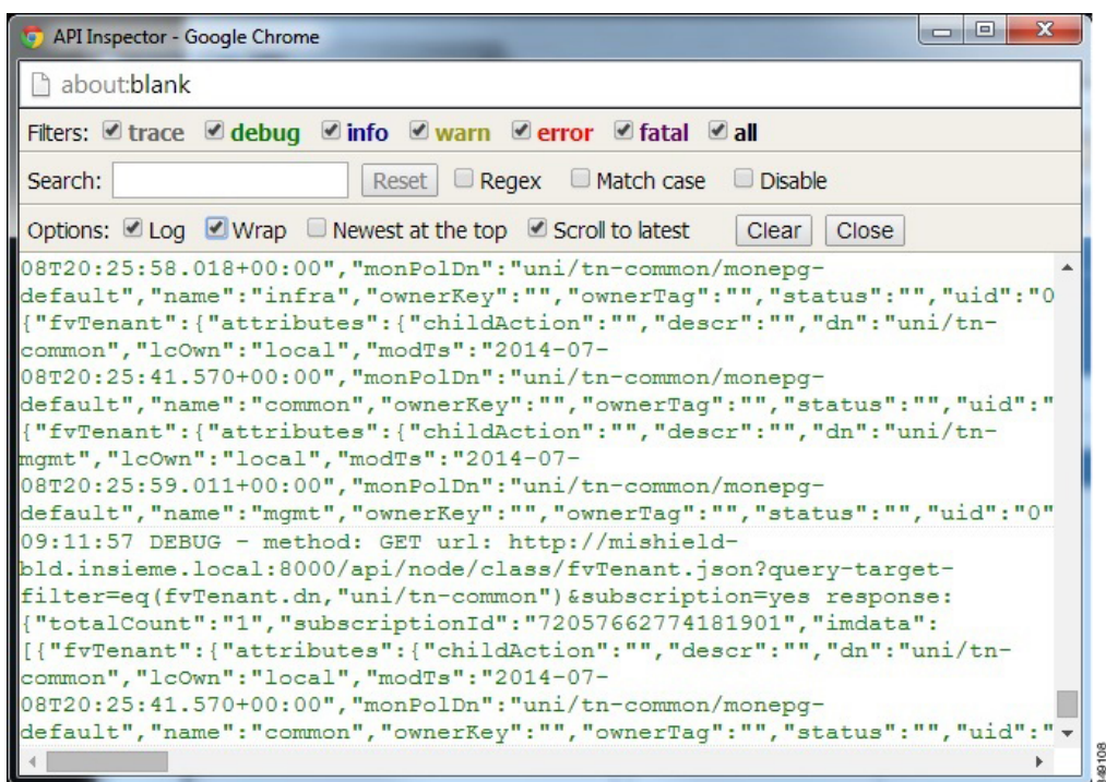
図 2: API インспекタ
