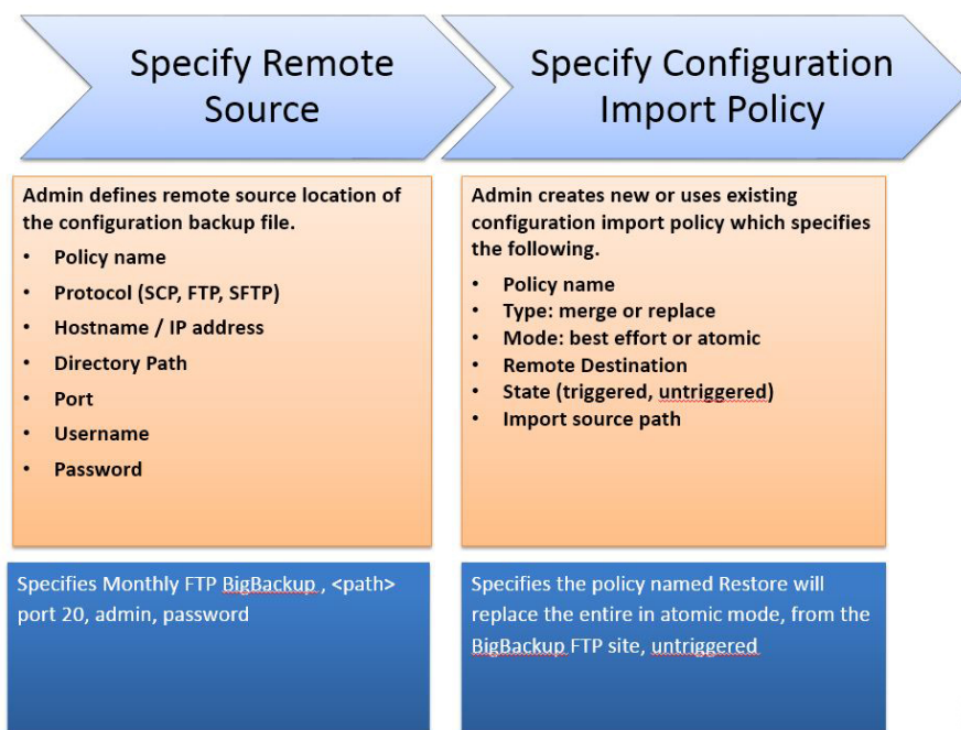
図 11: インポート ポリシーを構成するワークフロー
