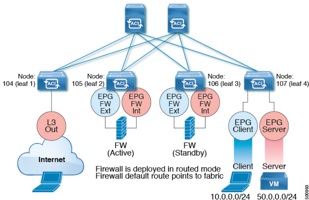
図 5: サンプルの ACI PBR 物理トポロジ
