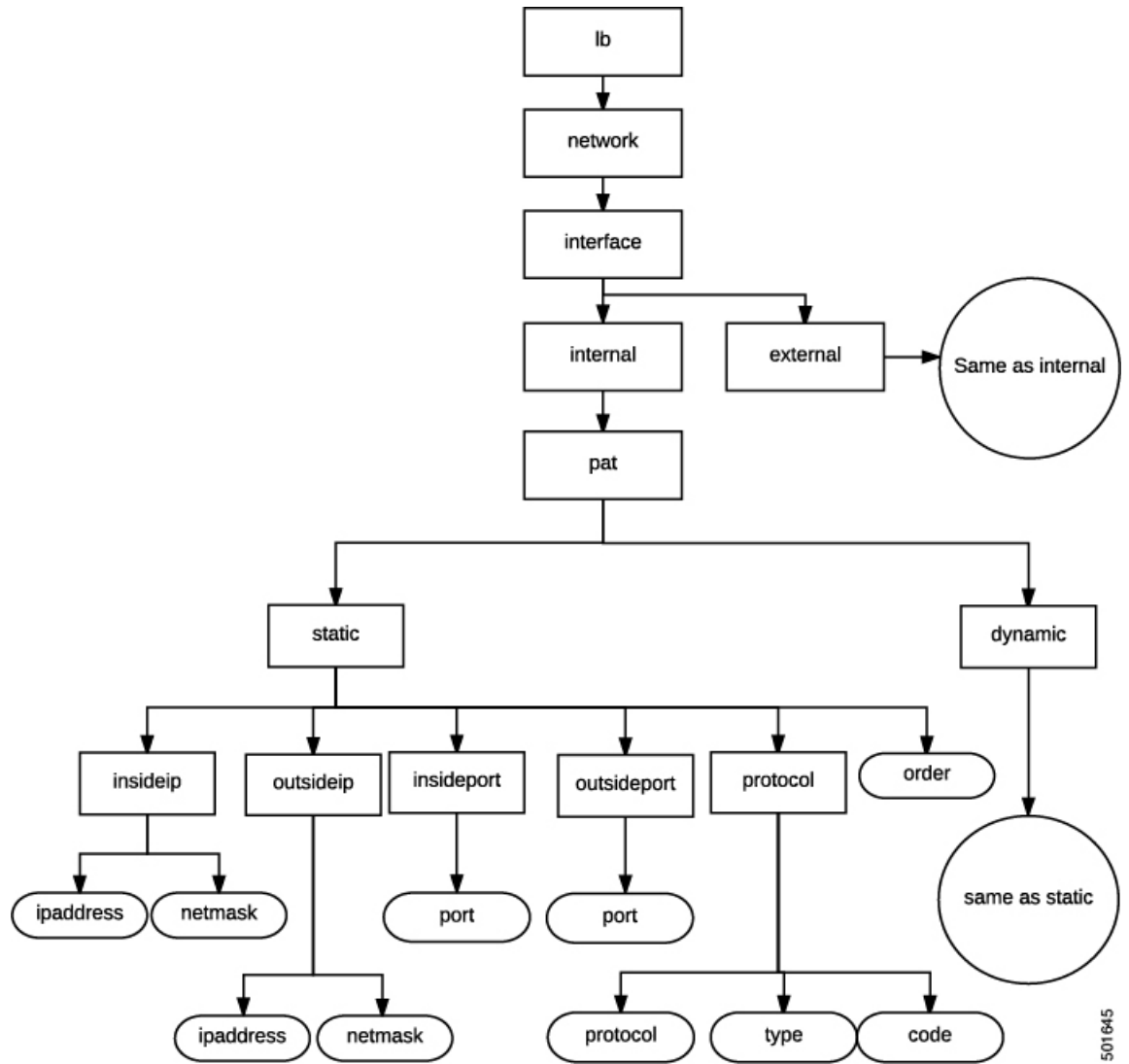
図 49: ロードバランサの PAT
