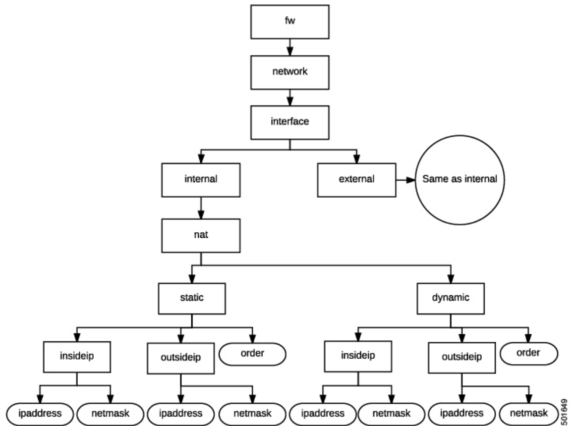
図 44: ファイアウォールの NAT
