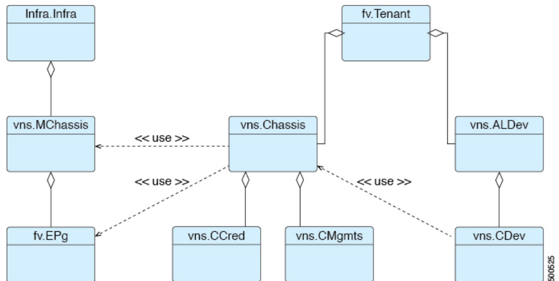
図 35: シャーシ マネージャのオブジェクト モデル
