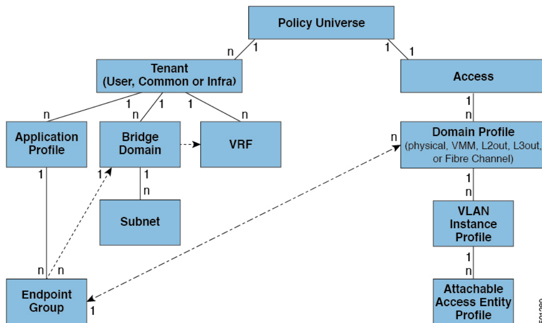
図 2: アクセスポリシーとエンドポイントグループの関連付け
