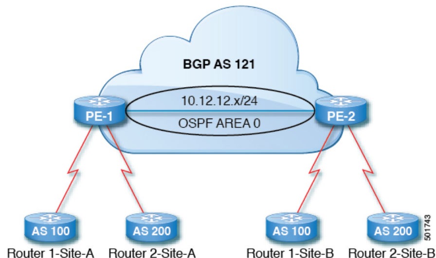
図 1: 自律システムオーバライド機能を説明するトポロジ例
