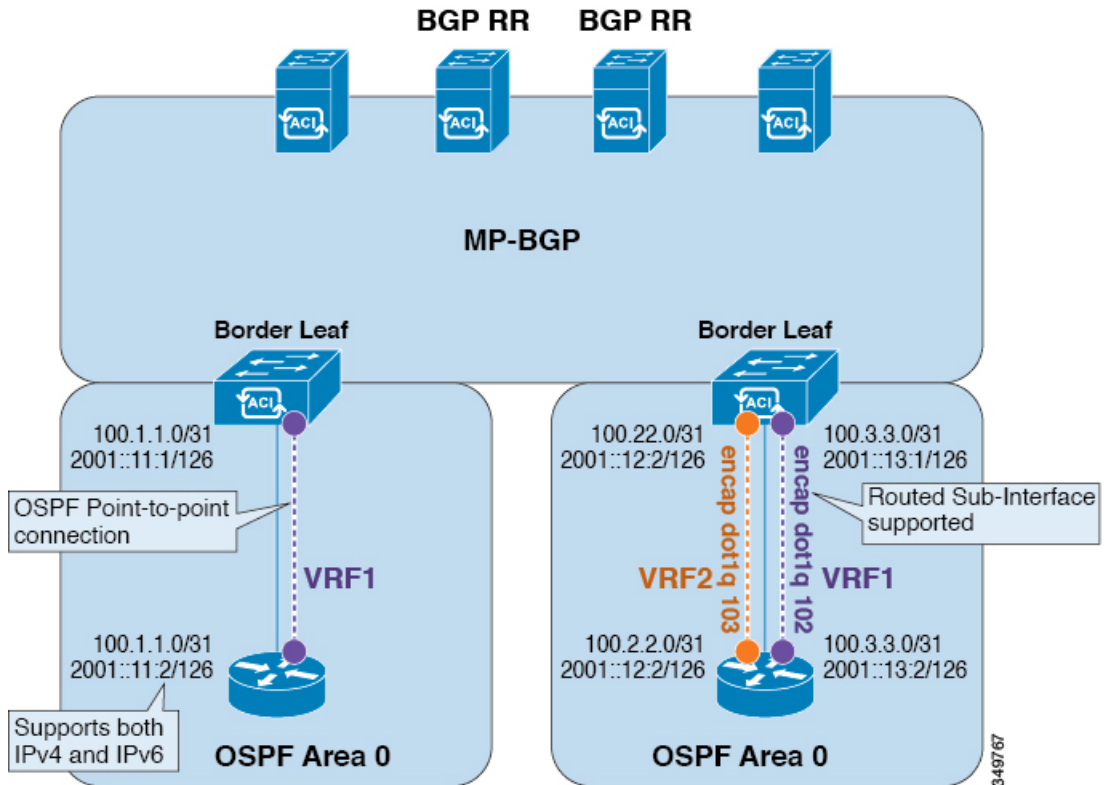
図 2: OSPF レイヤ 3 Out 接続
