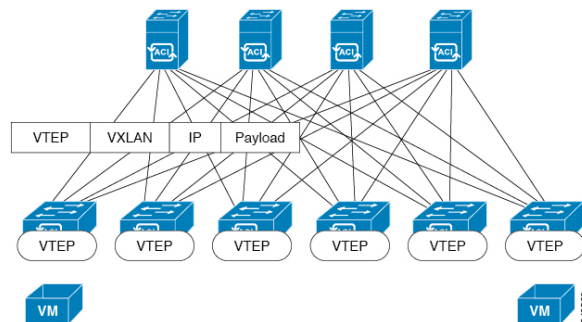
図 3: ACI によって切り離された ID と場所
