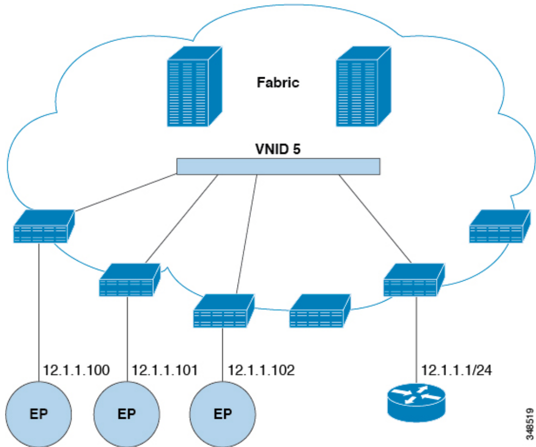
図 6: ブリッジ外部ルータ
