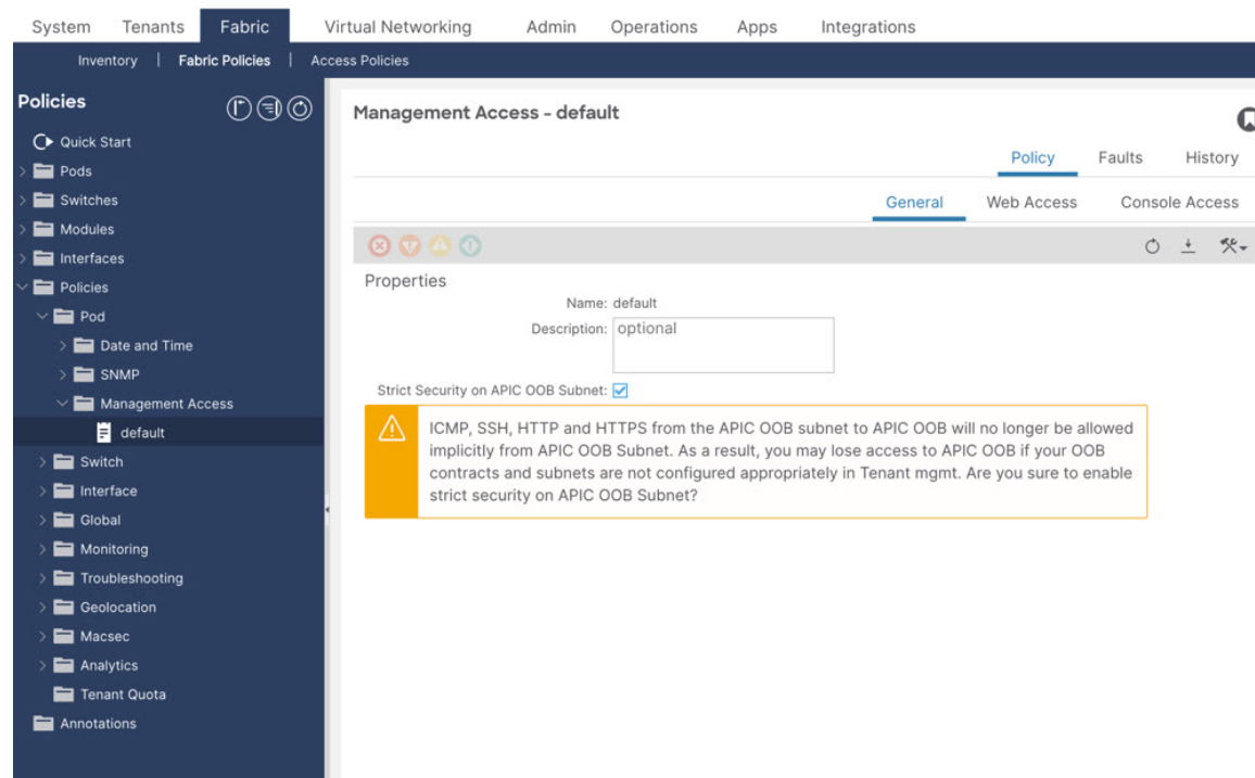
図 1: 厳密セキュリティ モードを有効にした後に表示される警告
