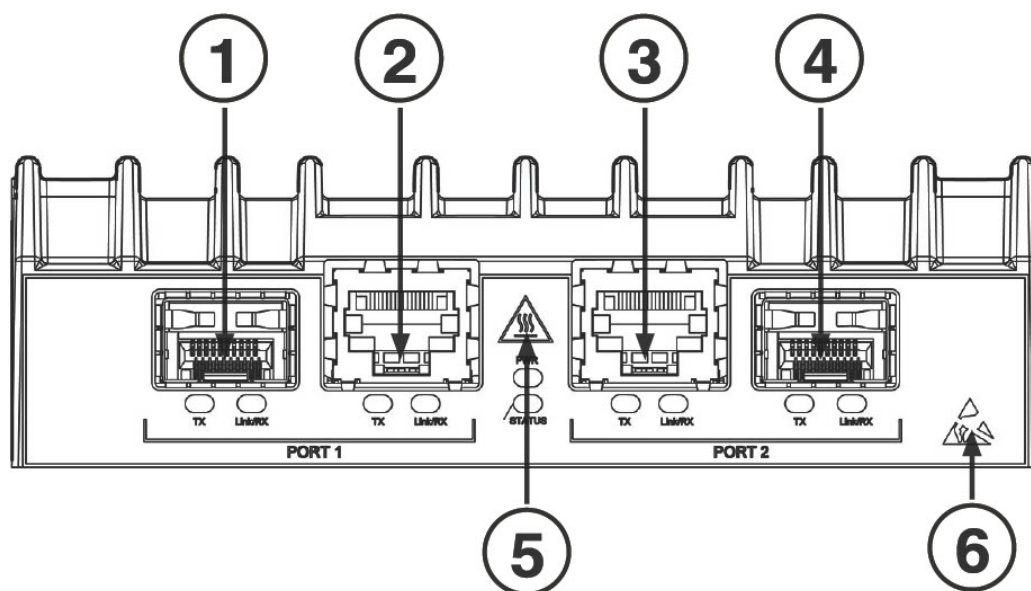
図 2: センサー モジュール 1G 前面パネル
