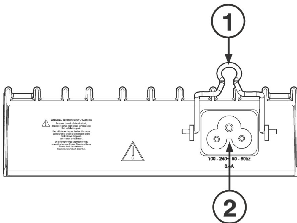
図 4: センサー モジュール 1G 背面パネル : AC 入力電源モデル
