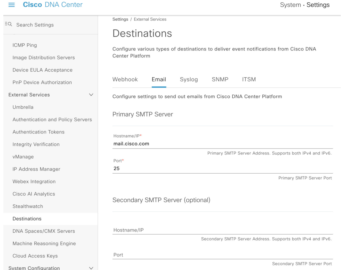
図 18: [Email] タブ
