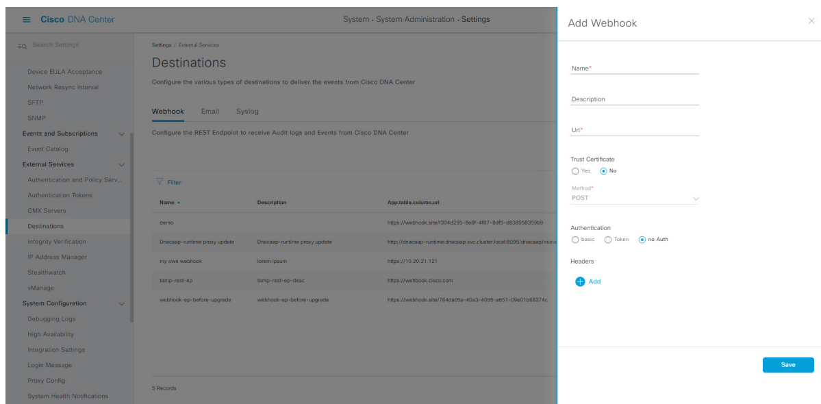
図 17: [Add Webhook]
