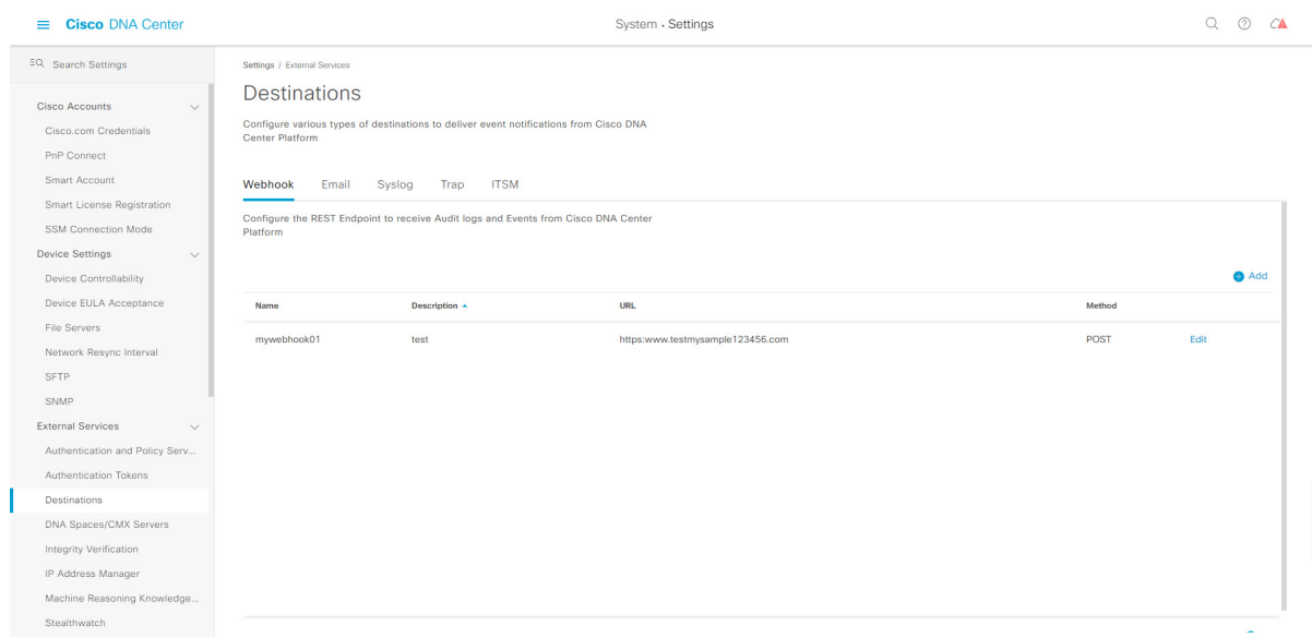
図 16 : [Webhook] タブ
