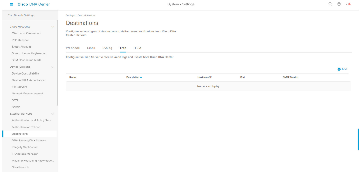
図 21:[Trap]タブ
