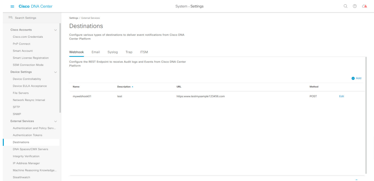
図 19: [Webhook] タブ
