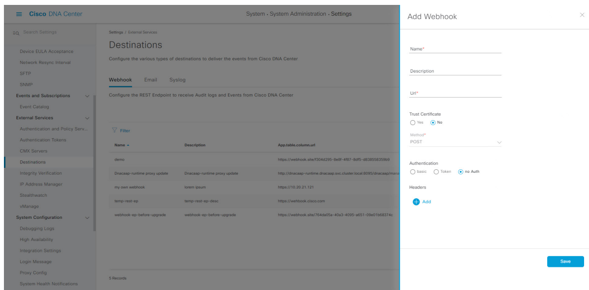
図 20: [Add Webhook]
