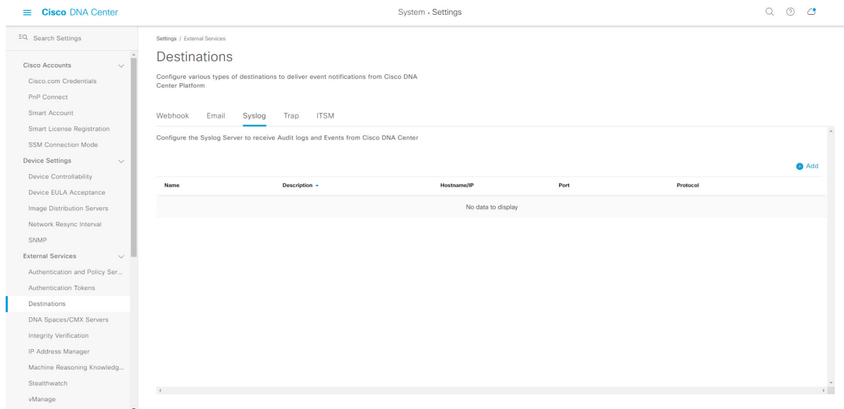
図 22 : [Syslog] タブ
