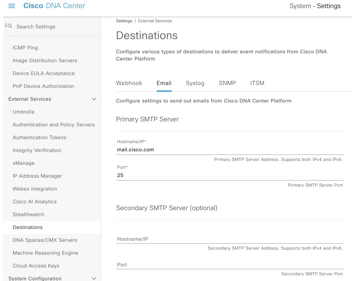
図 21 : [Email] タブ
