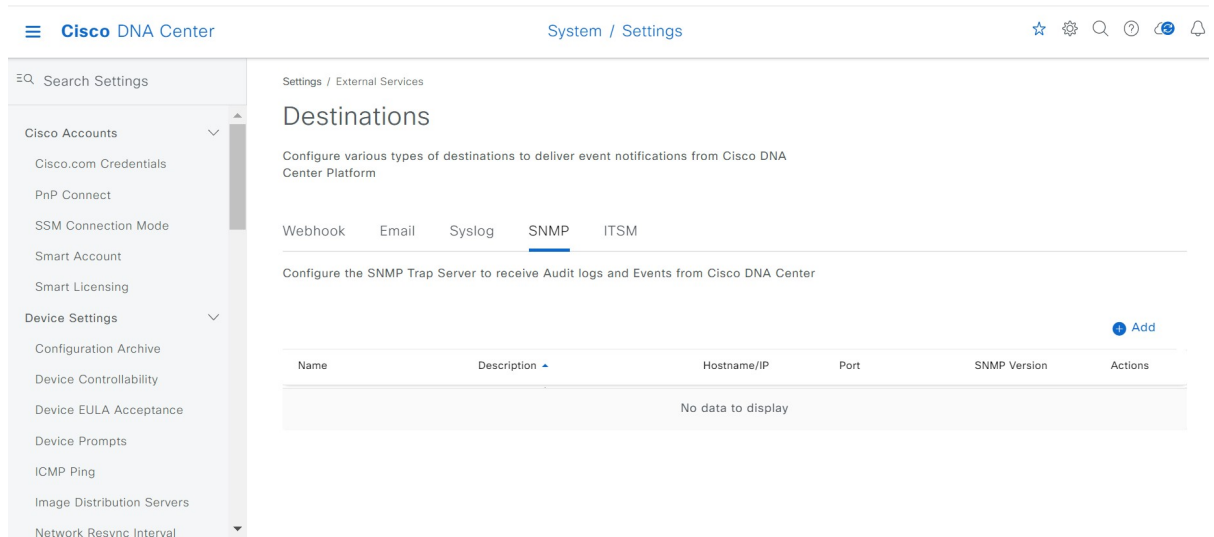
図 24: [Trap] タブ
