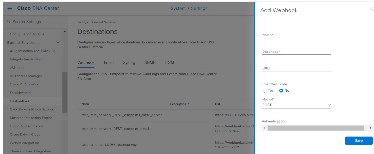
図 34 : [Add Webhook]
