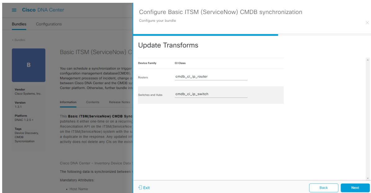
図 14: [Update Transforms] ウィンドウ
