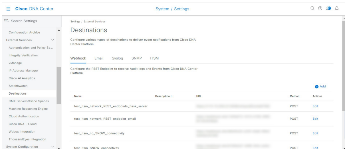
図 33: [Webhook] タブ
