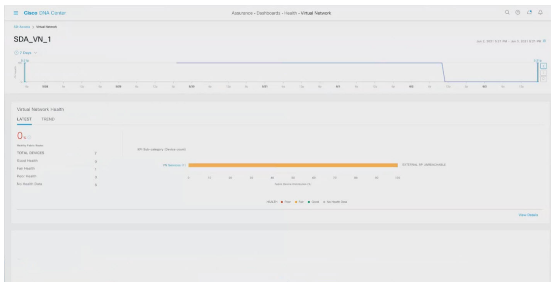
図 4: Virtual Network 360
