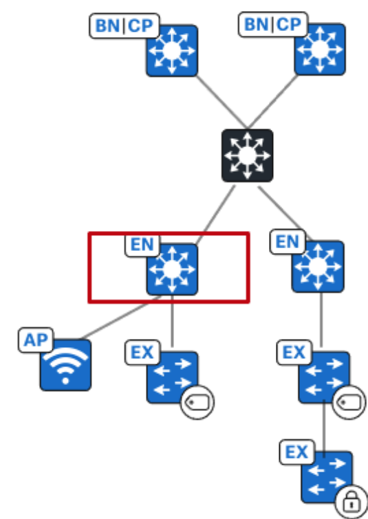
図 52. 障害が発生したファブリックエッジ (Switch-110-4-0-9) は、アップリンクの中間スイッチ (Switch-110-4-0-3) とダウンリンクの AP およびポリシー拡張ノードに接続されています。
