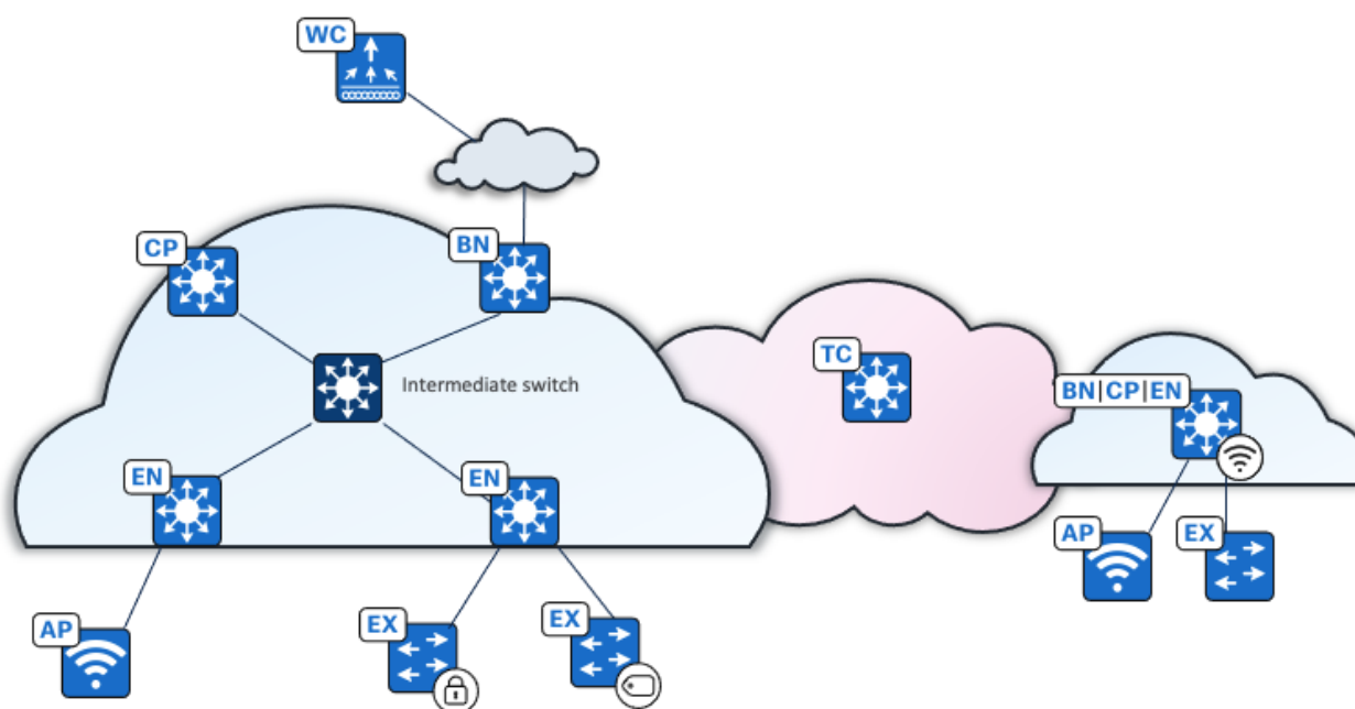
図 8. ファブリックロール
