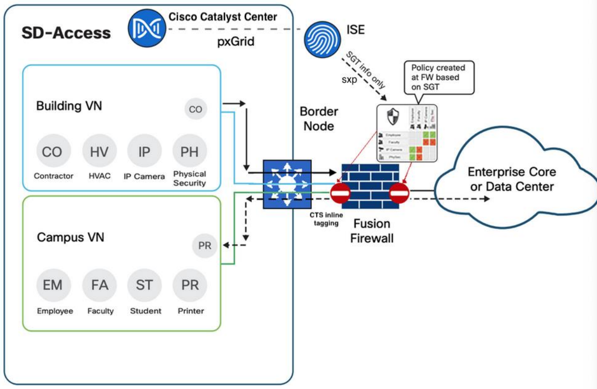
図 18. Cisco SD-Access の導入における一般的なファイアウォール機能
