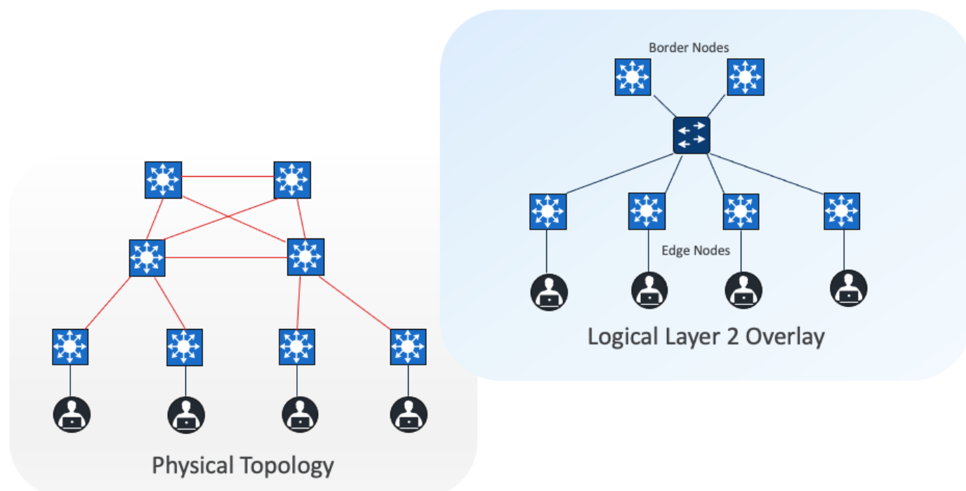
図 3. 論理的に接続がスイッチされるレイヤ 2 オーバーレイ
