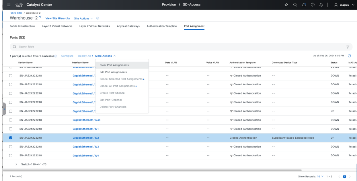
図 64. SBEN がインベントリから削除された後のアップリンクデバイス上での物理ポート設定の削除
