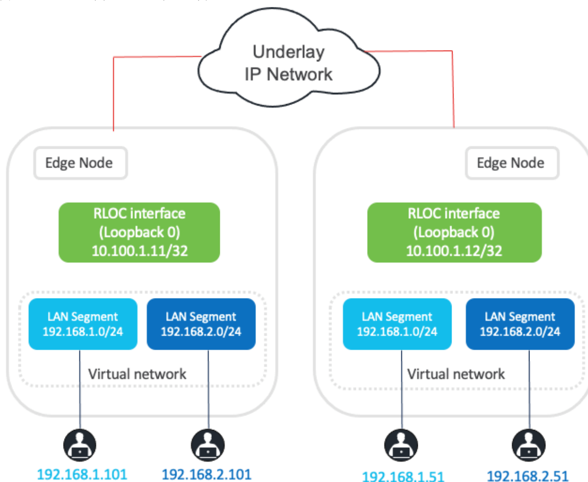
図 5. サブネットストレッチの例
