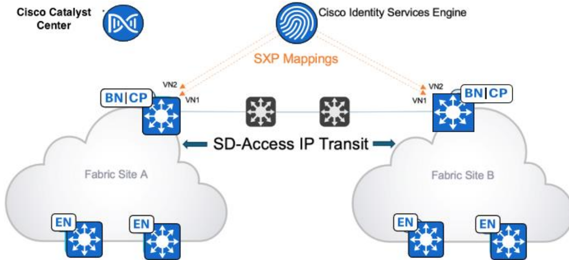
図 17. リモートボーダーへの SXP マッピングの送信
