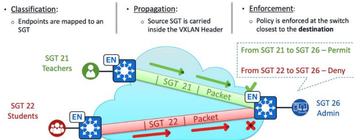
図 15. エンドポイントトラフィックの Cisco SD-Access の展開におけるマイクロセグメンテーションの仕組み
