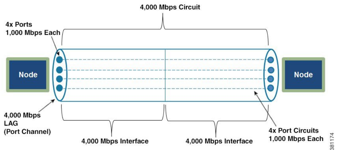
図 1: ポート、ポート回線、および LAG
