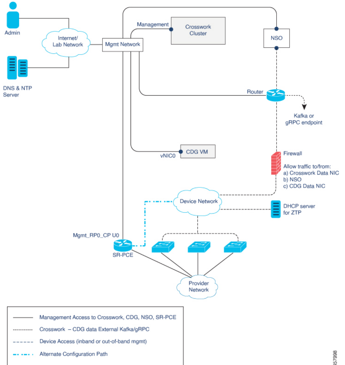
図 1: Cisco Crosswork : 1 NIC ネットワークポロジ
