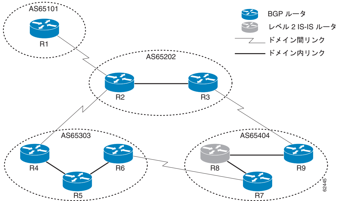
図 3 汎用 BGP CLNS ネットワークのコンポーネント
