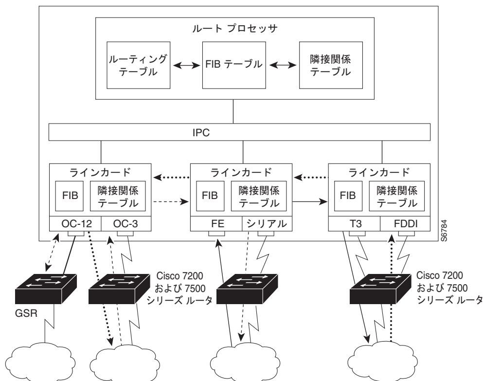
図 2 分散型シスコ エクスプレス フォワーディング モードの動作
