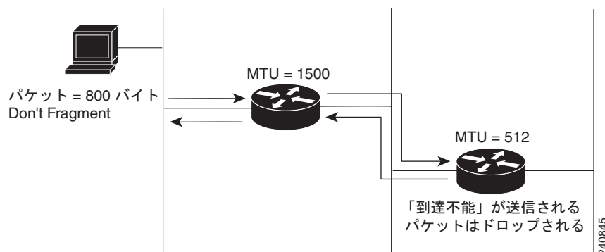
図 1 IP PMTUD
