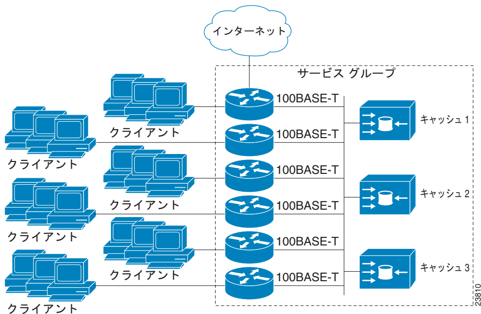
図 2 WCCPv2 を使用する Cisco Cache Engine のネットワーク設定
