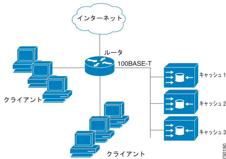
図 1 WCCPv1 の設定
