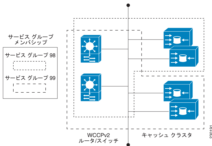
図 3 WCCP サービス グループ
