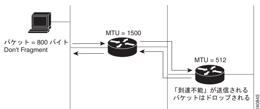
図 1 IP PMTUD
