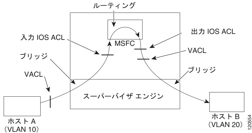
図 37-2 ルーティング対象パケットへの VACL の適用
