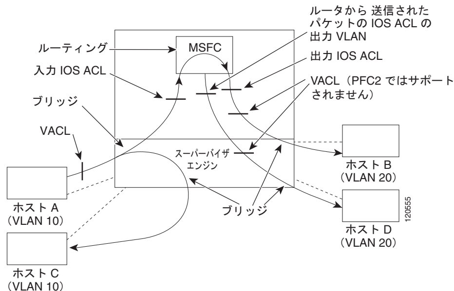
図 37-3 マルチキャスト パケットへの VACL の適用
