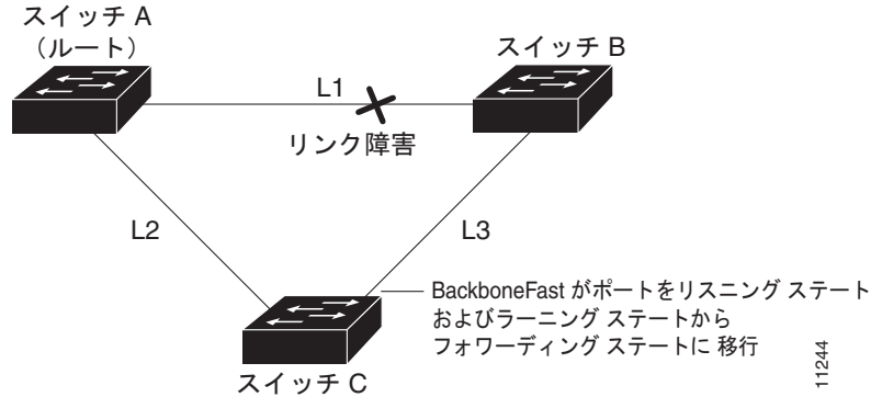
図 21-4 間接リンク障害が発生したあとの BackboneFast の例
