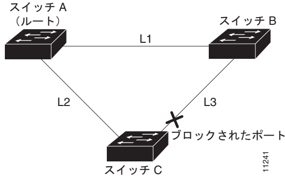
図 21-1 直接リンク障害が発生する前の UplinkFast の例
