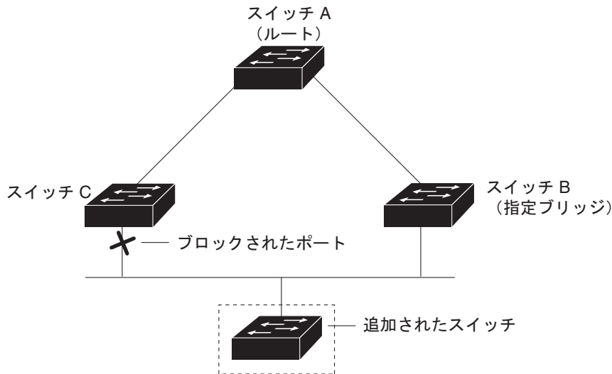
図 21-5 メディア共有型トポロジーにおけるネットワーク デバイスの追加
