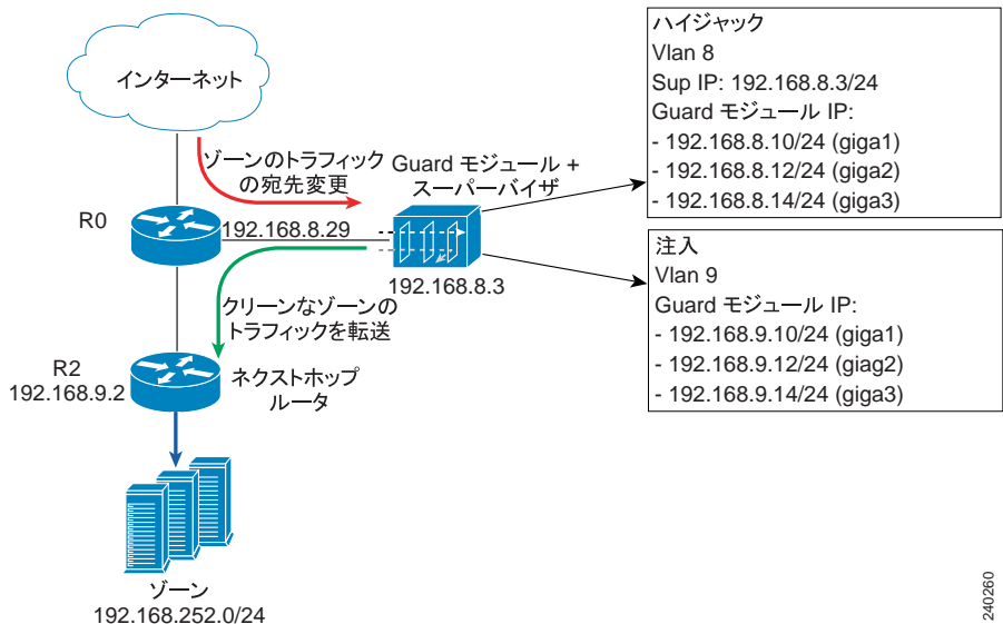
図 5-5 レイヤ 3 トポロジを持つアウトオブパス ネットワーク設定のサンプル (3 Gbps 動作)
