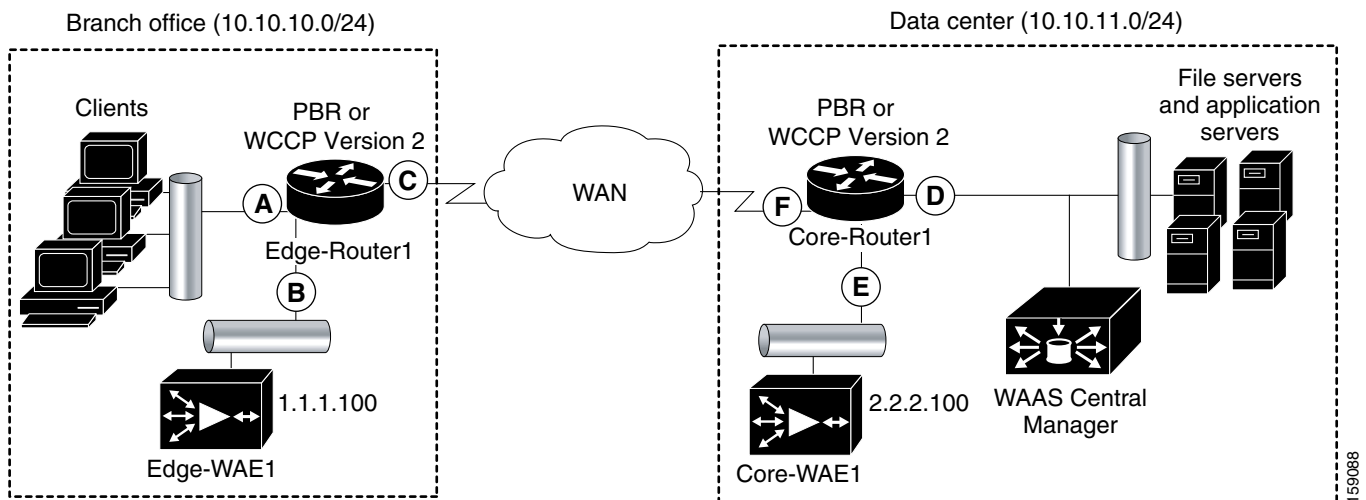
図 2-1 PBR または WCCP バージョン 2 を使用してすべての TCP トラフィックを透過的に WAE へリダイレクトする
