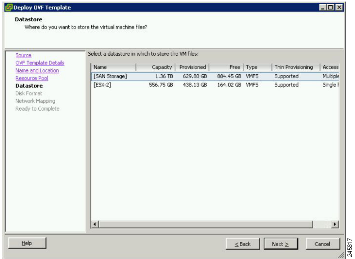
図 4 vWAAS : データストア
