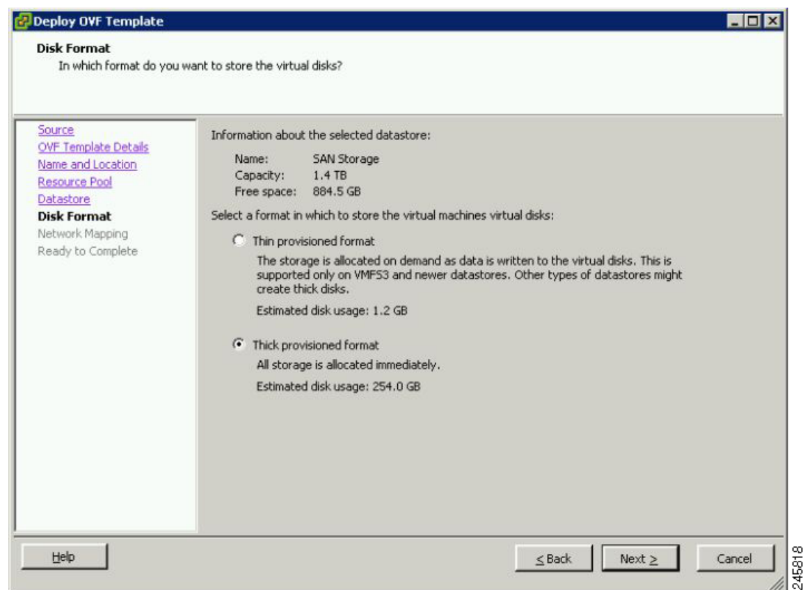
図 5 vWAAS : ディスク フォーマット
