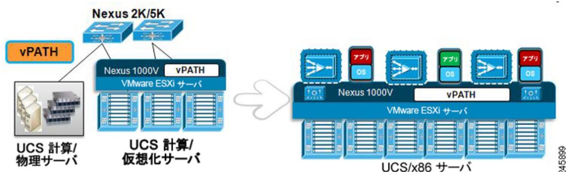
図 11 vWAAS : vPATH インターセプション
