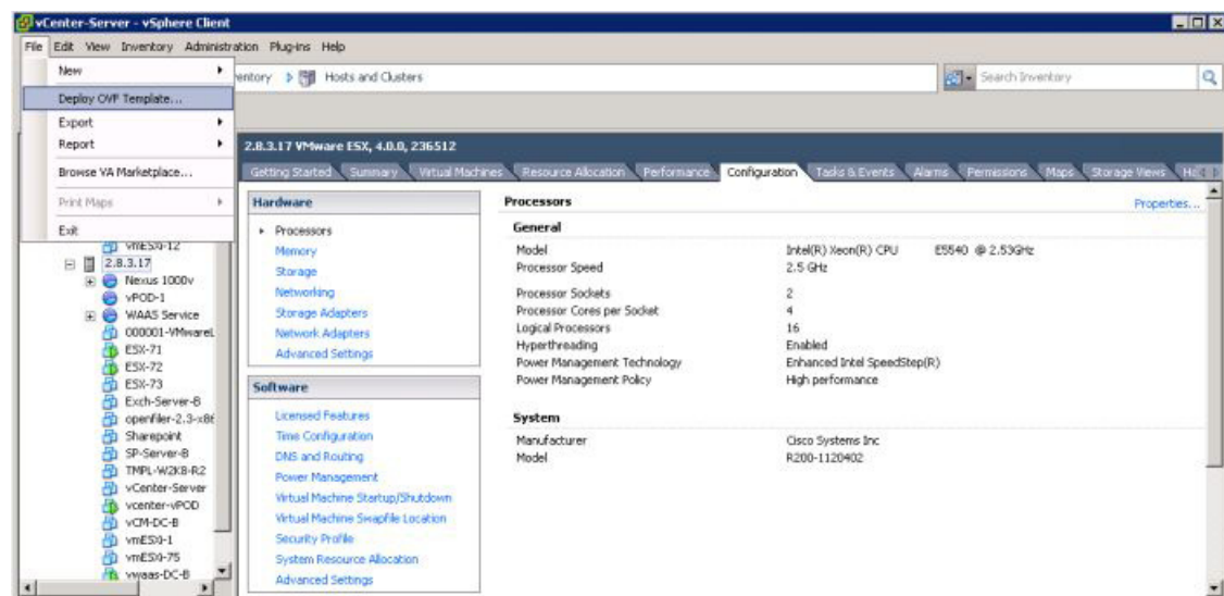
図 2 vWAAS : OVF テンプレートの展開
