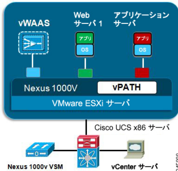
図 10 vPATH インターセプションの概要
