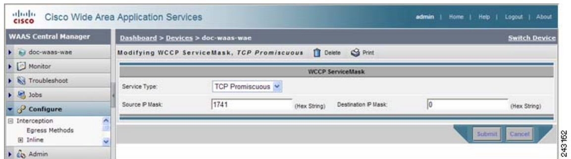
図 4-4 WCCP サービス マスクの変更
