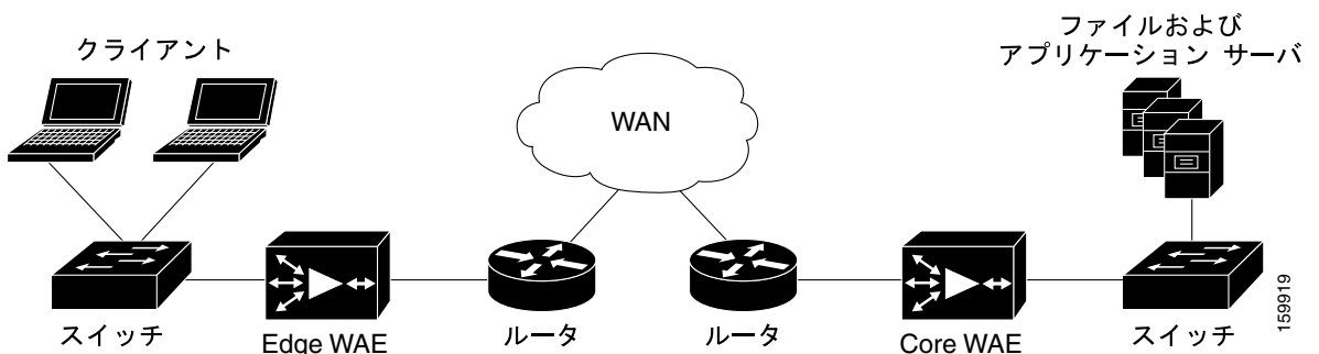
図 4-8 インライン代行受信
