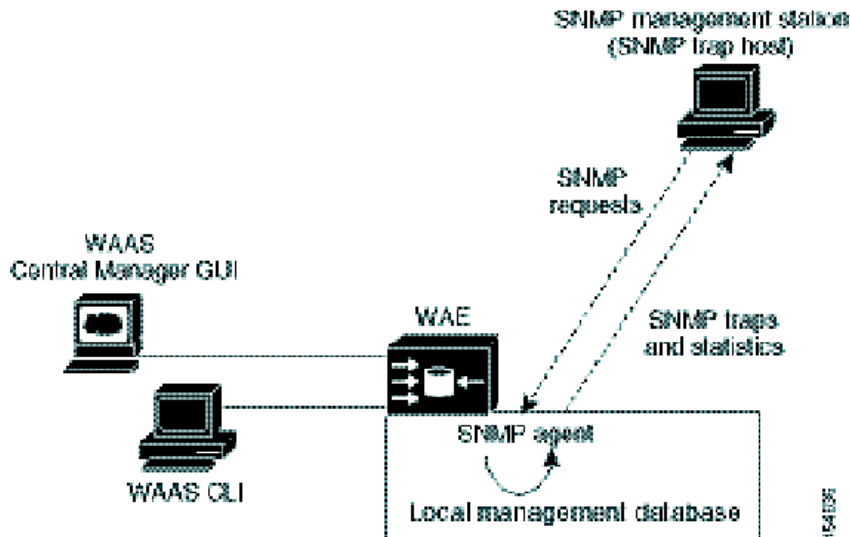
図 17-1 WAAS ネットワーク内の SNMP コンポーネント
