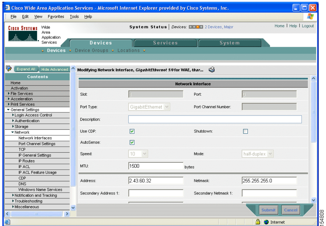
図 5-1 [Modifying Network Interface] ウィンドウ — スタンバイ グループ優先順位設定
