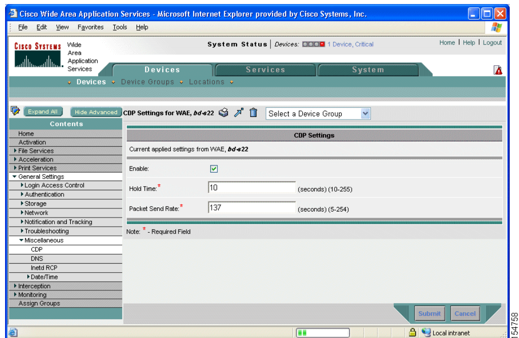
図 5-3 [CDP Settings] ウィンドウ
