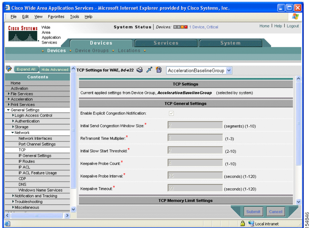
図 5-2 [TCP Settings] ウィンドウ
