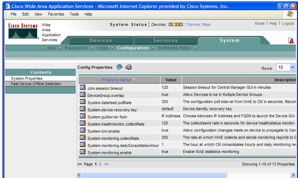
図 9-3 [Config Properties] ウィンドウ
