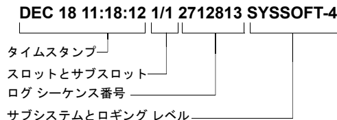
図 4-2 ログ メッセージのロギング ヘッダー
