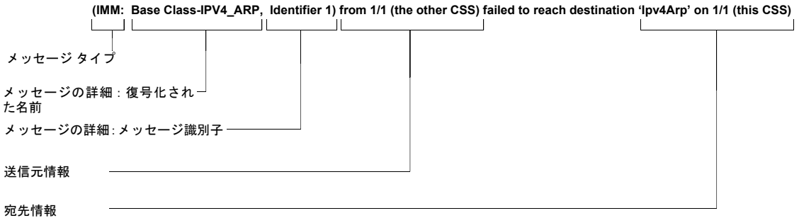
図 4-4 ロギングメッセージのフィールド
