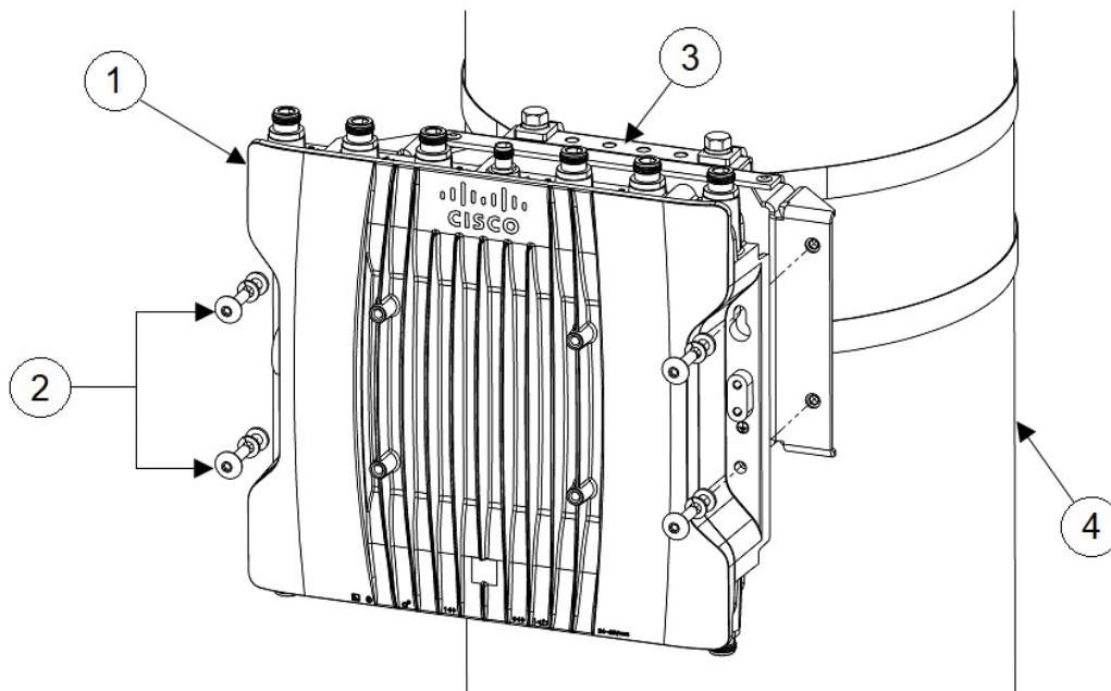
図 12: 取り付けブラケットに取り付けたアクセス ポイント
