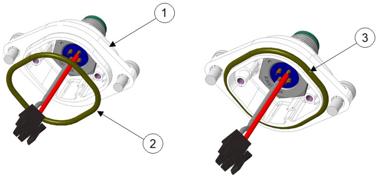
図 16: M12 アダプタへの O リングの取り付け
