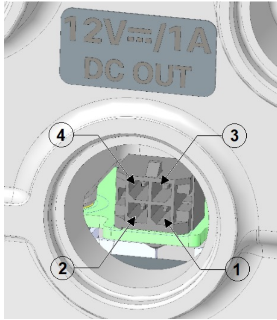
図 11: 12V/1A DC 出力ポート
