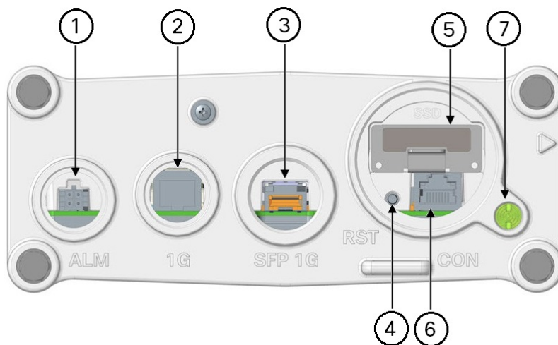
図 3: CPU モジュールコンポーネント
