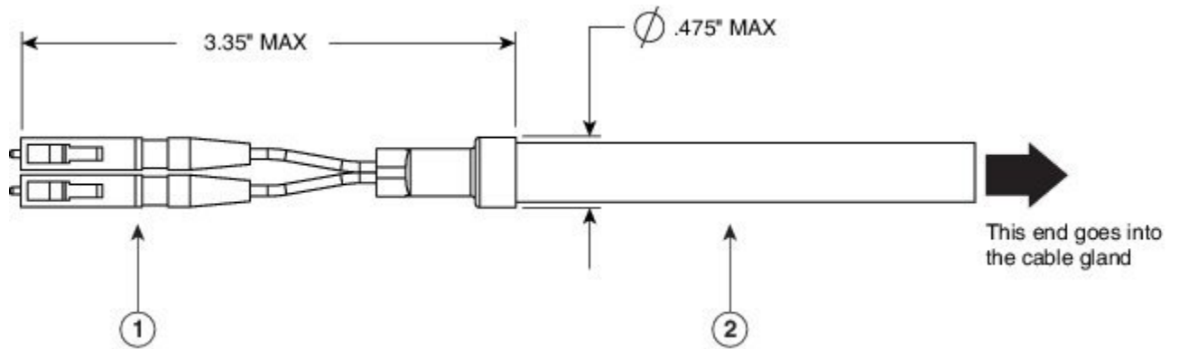
図 7:デュプレックス LC 光ファイバ ケーブル
