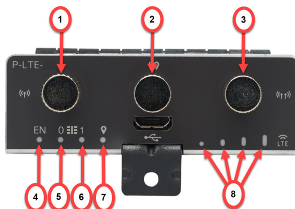
図 1: LTE プラガブルモジュール (前面)
