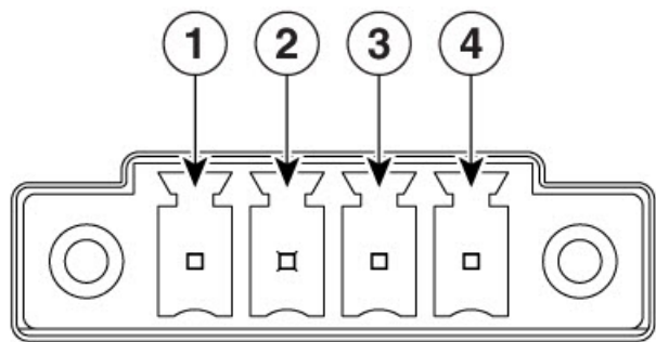
図 1: 電源コネクタのピン配置
