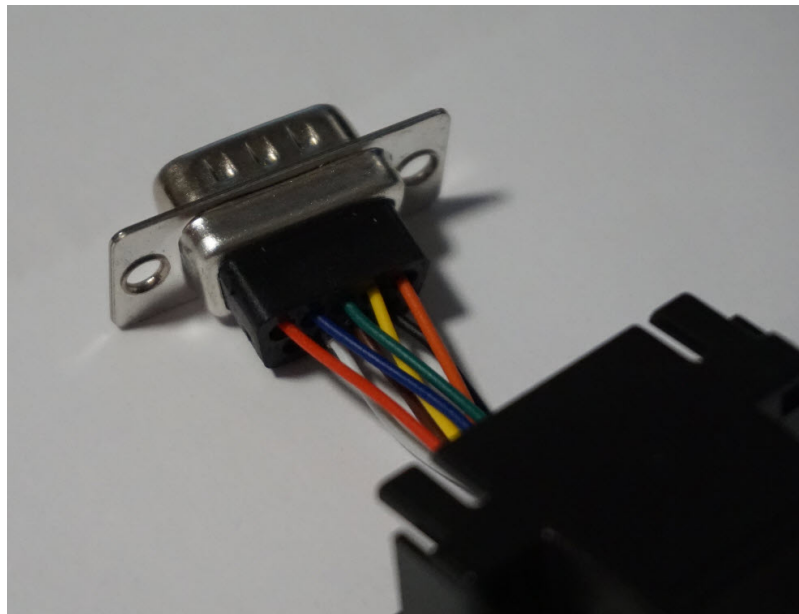
図 7: 完了したピン接続
