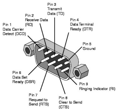
図 3: RS-232 DB9 オスコネクタのオス側からのビュー
