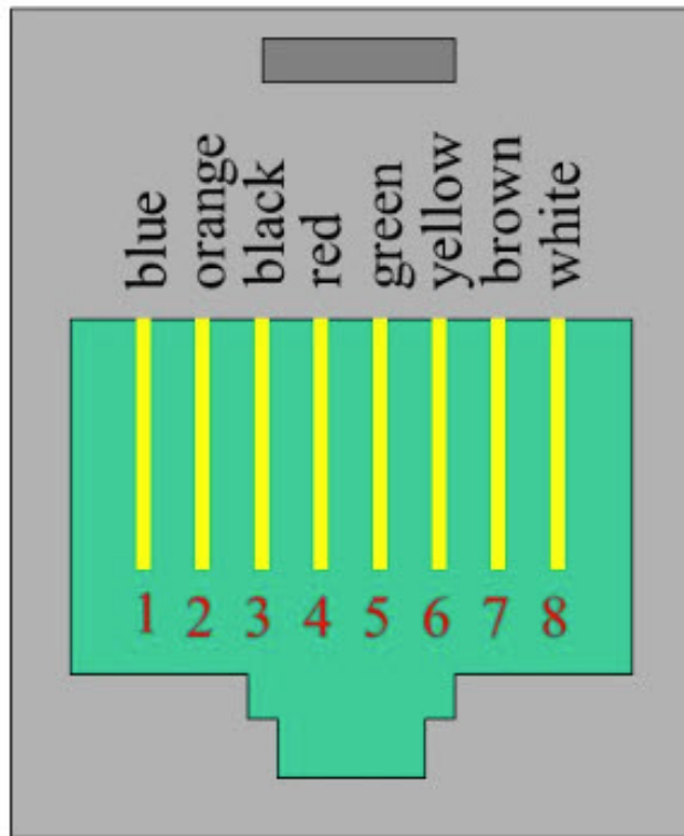
図 5: RJ-45 メス側ピン割り当て
