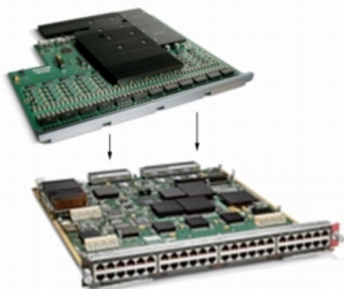
図 6 802.3af PoE ドーターカード ( 上 ) ( 製品番号 WS-F6K-GE48-AF ) を搭載した Cisco クラシック 48 ポート 10/100/1000 モジュール ( 製品番号 WS-X6148A-GE-TX )
