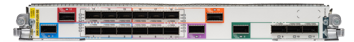
図 1. Cisco ASR 9000 シリーズ 2T サービス エッジ コンボ ライン カード : 第 5 世代 : SE
