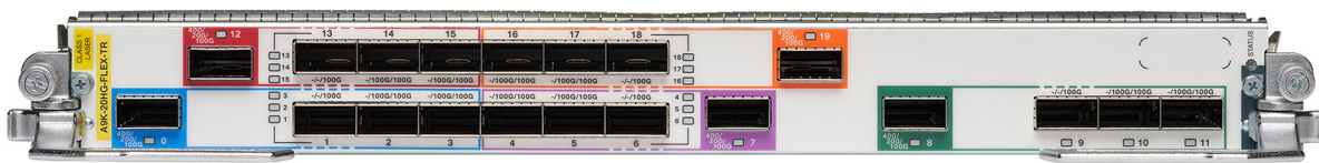
図 2. Cisco ASR 9000 シリーズ 2T パケット トランスポート コンボ ライン カード : 第 5 世代 : TR
