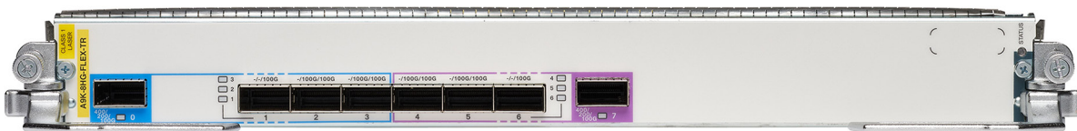
図 4. Cisco ASR 9000 シリーズ 800G パケット トランスポート コンボ ライン カード : 第 5 世代 : TR
